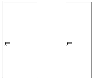
ID-01 10 x21M LYD: 0dB R'w ID-02 8 x21M LYD: 0dB R'w
