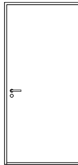
IDK01 10 x21M BRANN: EI30 LYD: 40dB R'w
