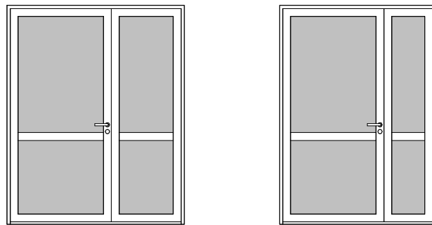
IDB40 17 x21M BRANN: EI30 IDB41 15 x21M BRANN: EI30
