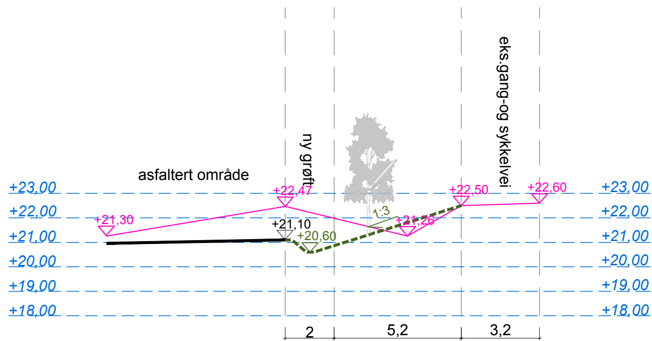
Terrengsnitt FF' 1:150
