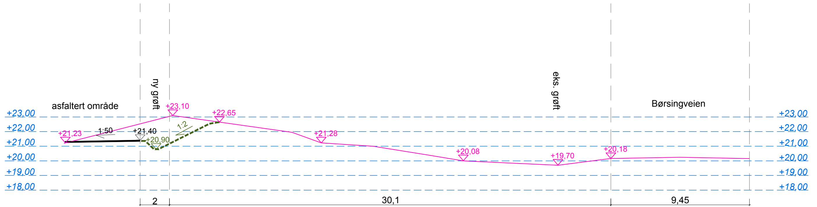
Terrengsnitt EE' 1:150
