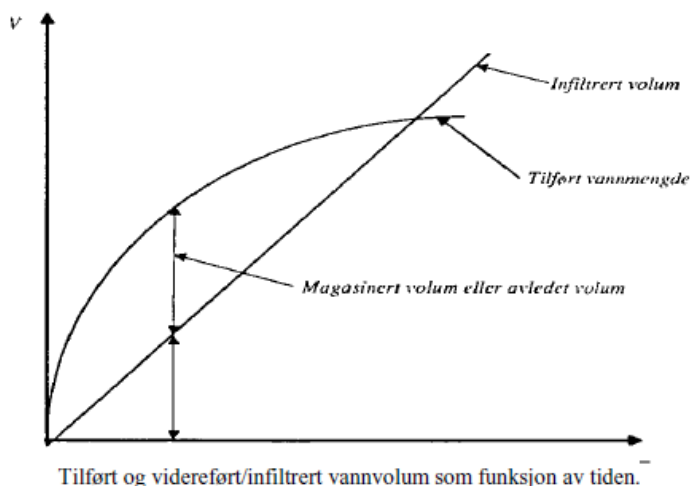
Figur 8: Prinsipp for å bestemme nødvendig fordrøyningsvolum
