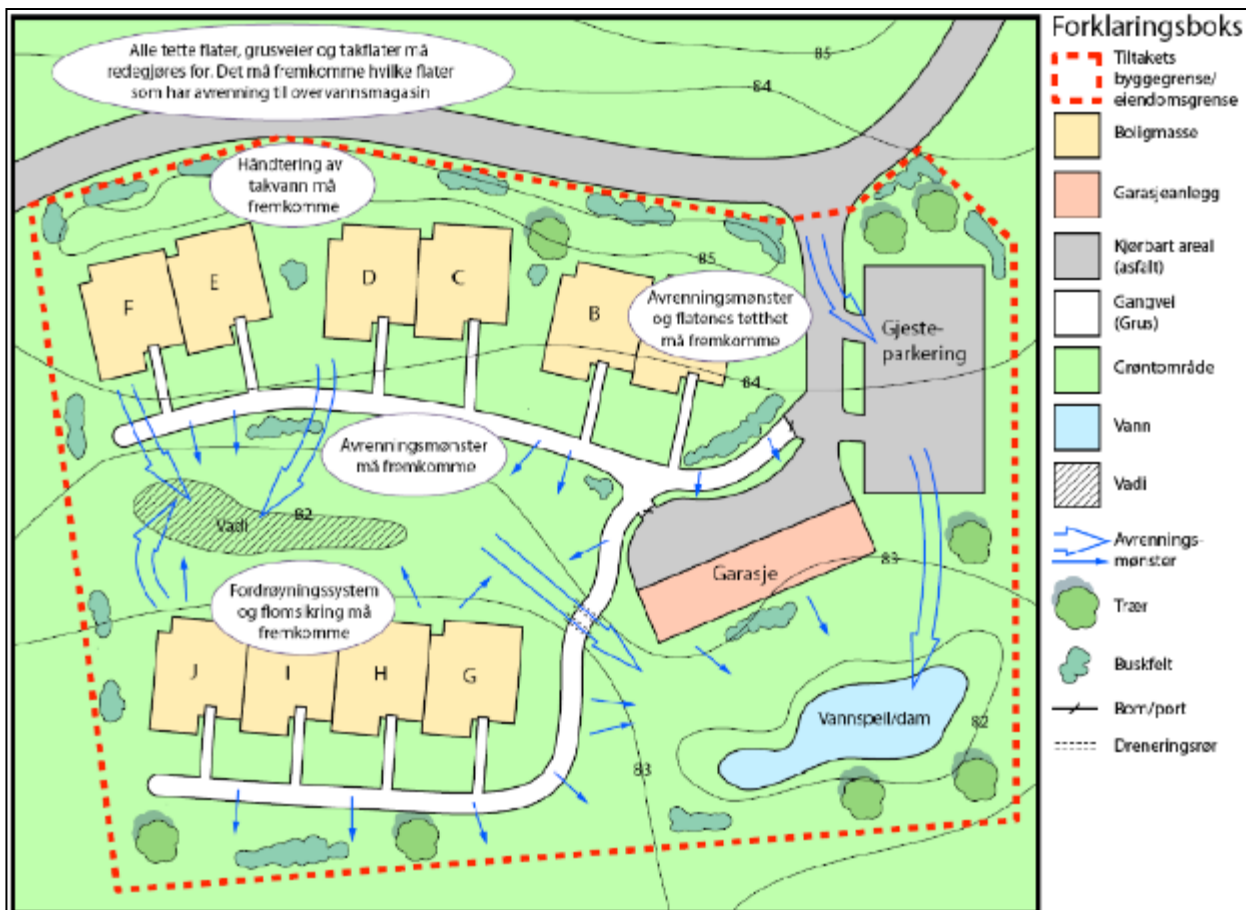
Figur 7: Eksempel på utomhusplan (kilde: Overvannshåndtering – En veileder for utbygger, Oslo kommune)
