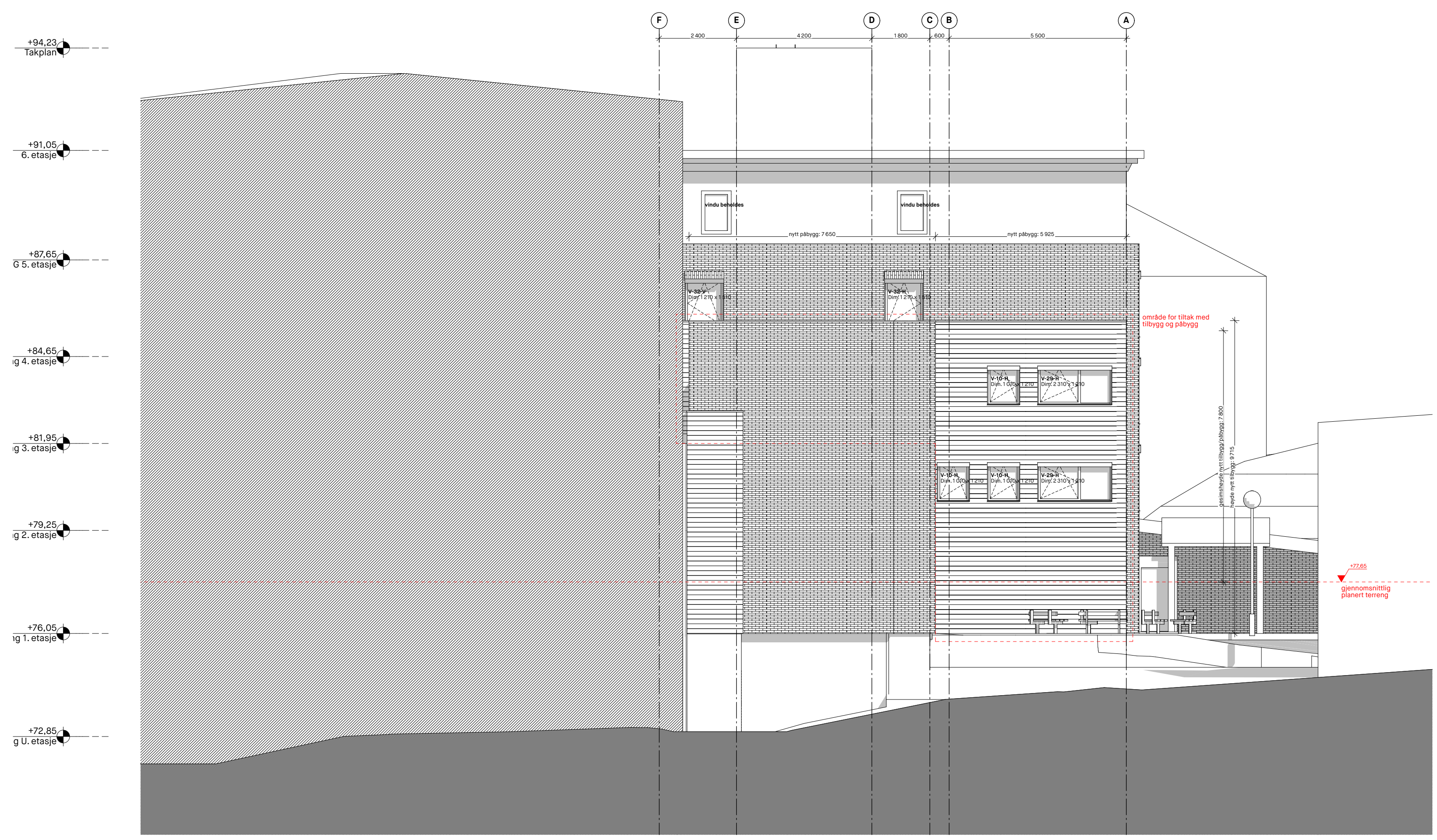
Fasade Nord etter tiltak 1:100
