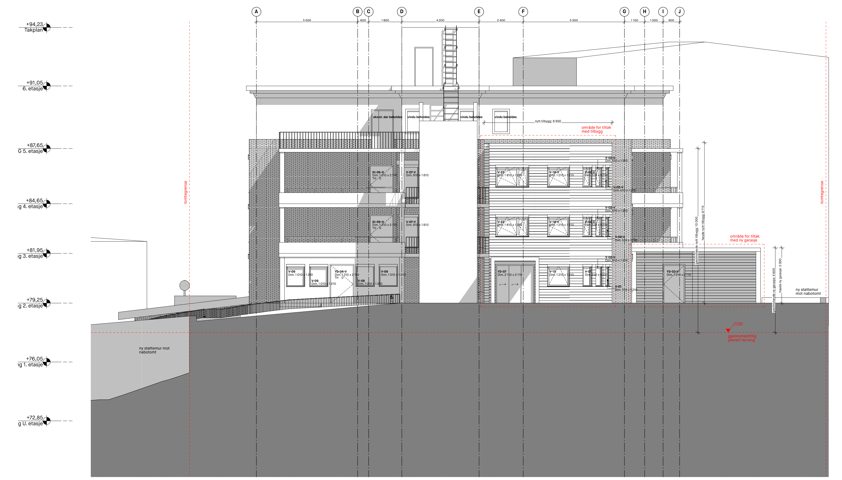
Fasade Sør etter tiltak 1:100
