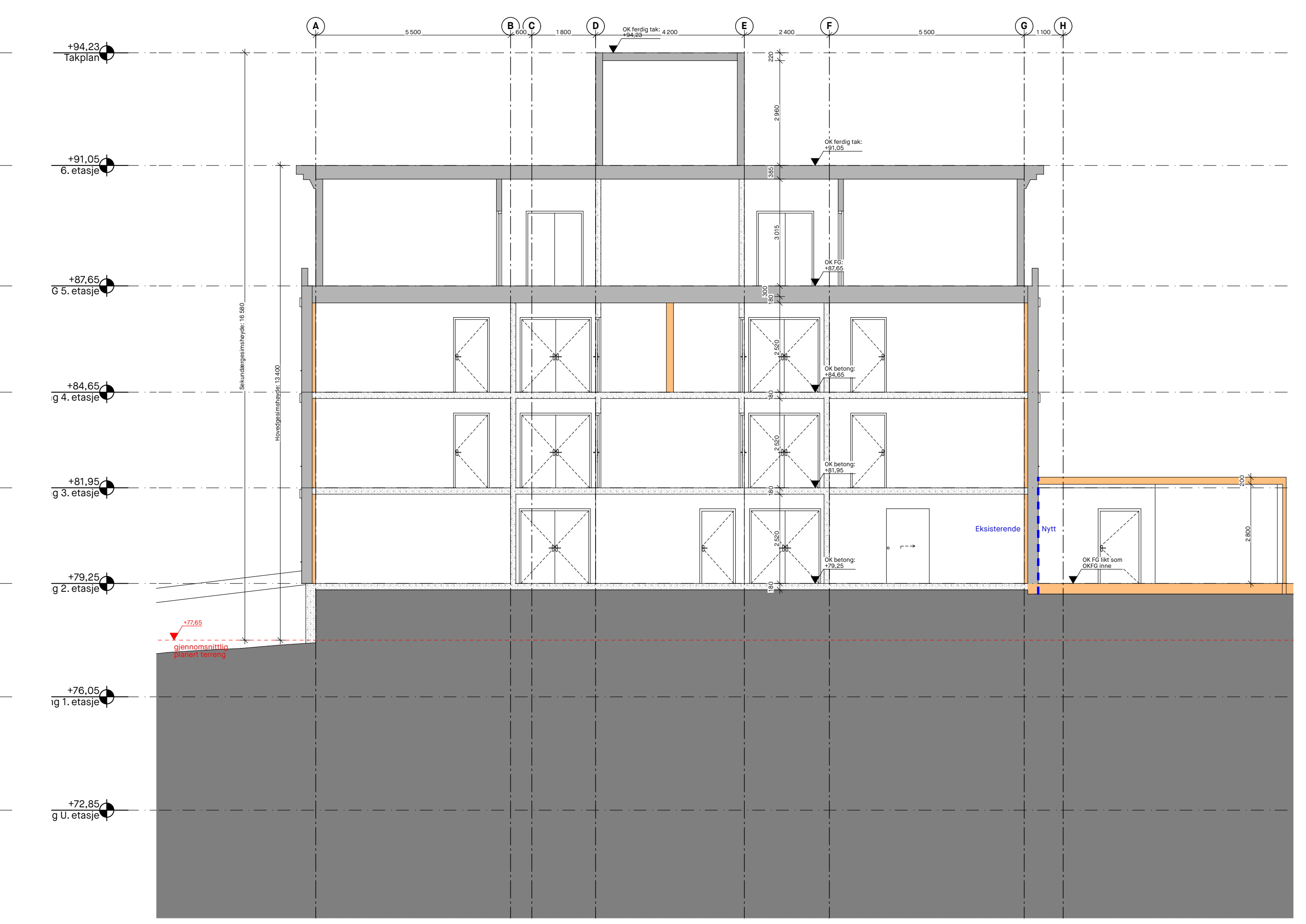
Snitt C etter tiltak 1:100
