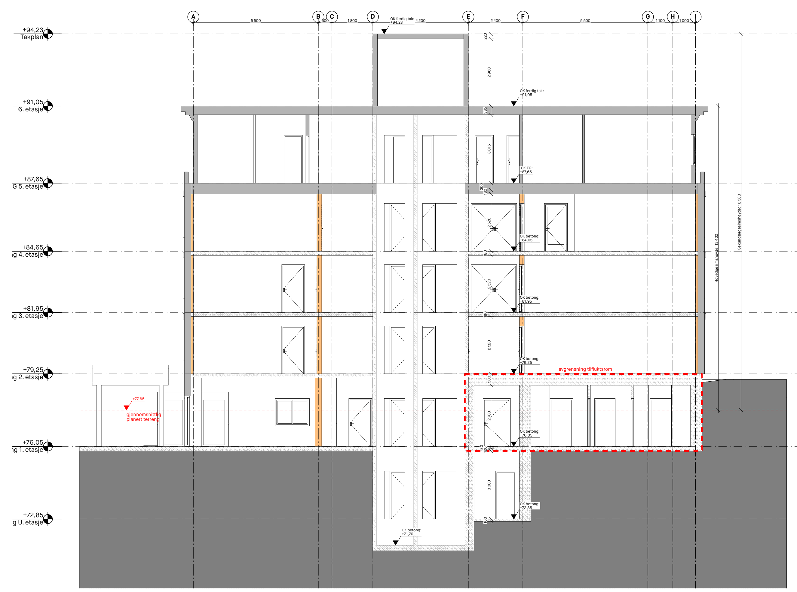
Snitt B etter tiltak 1:100
