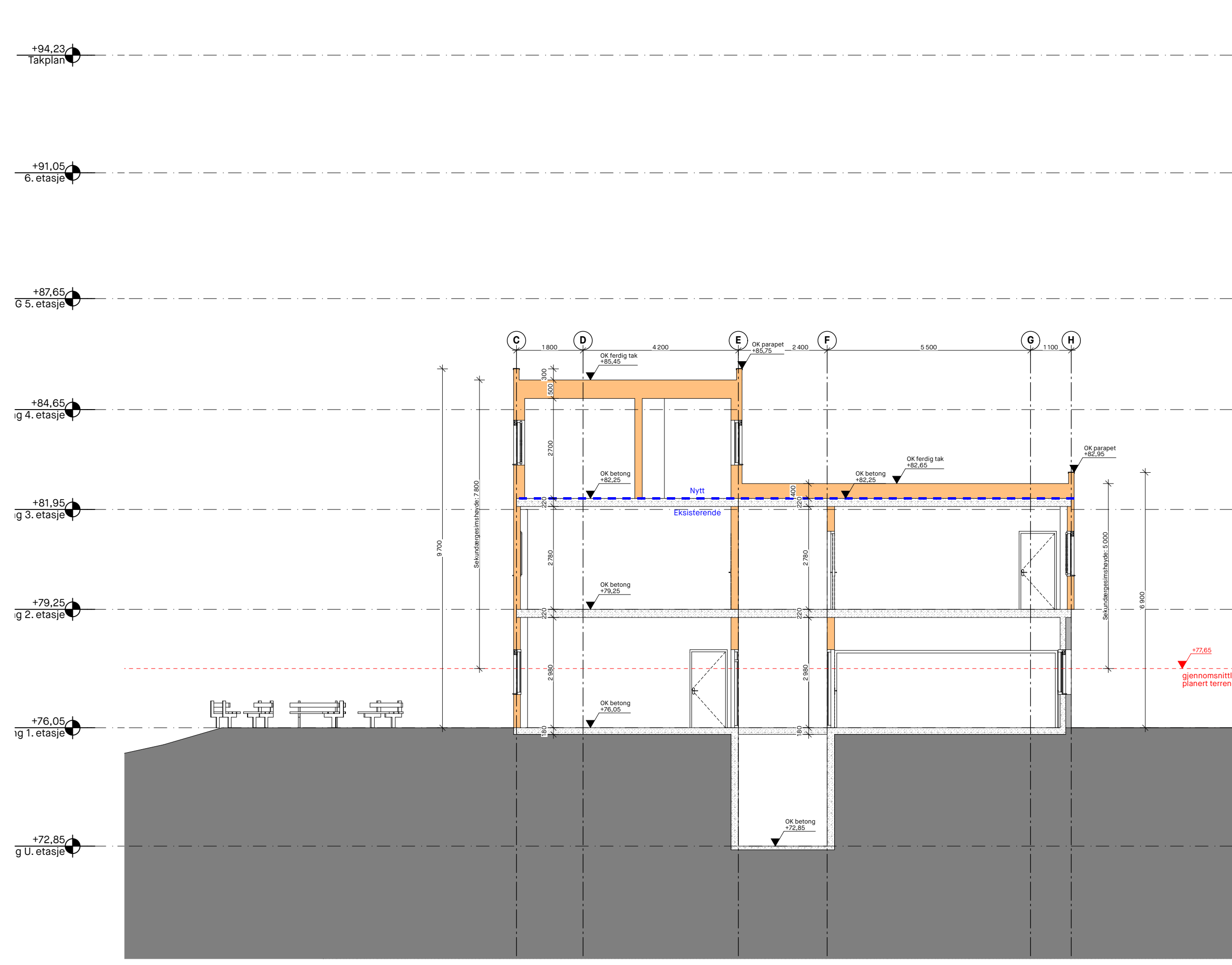
Snitt A etter tiltak 1:100
