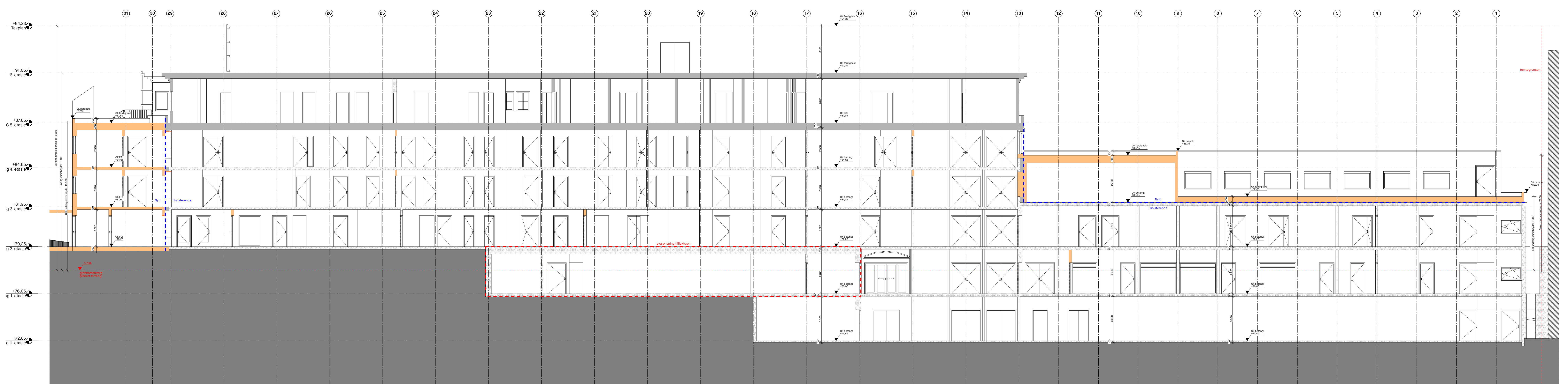
Snitt E etter tiltak 1:100
