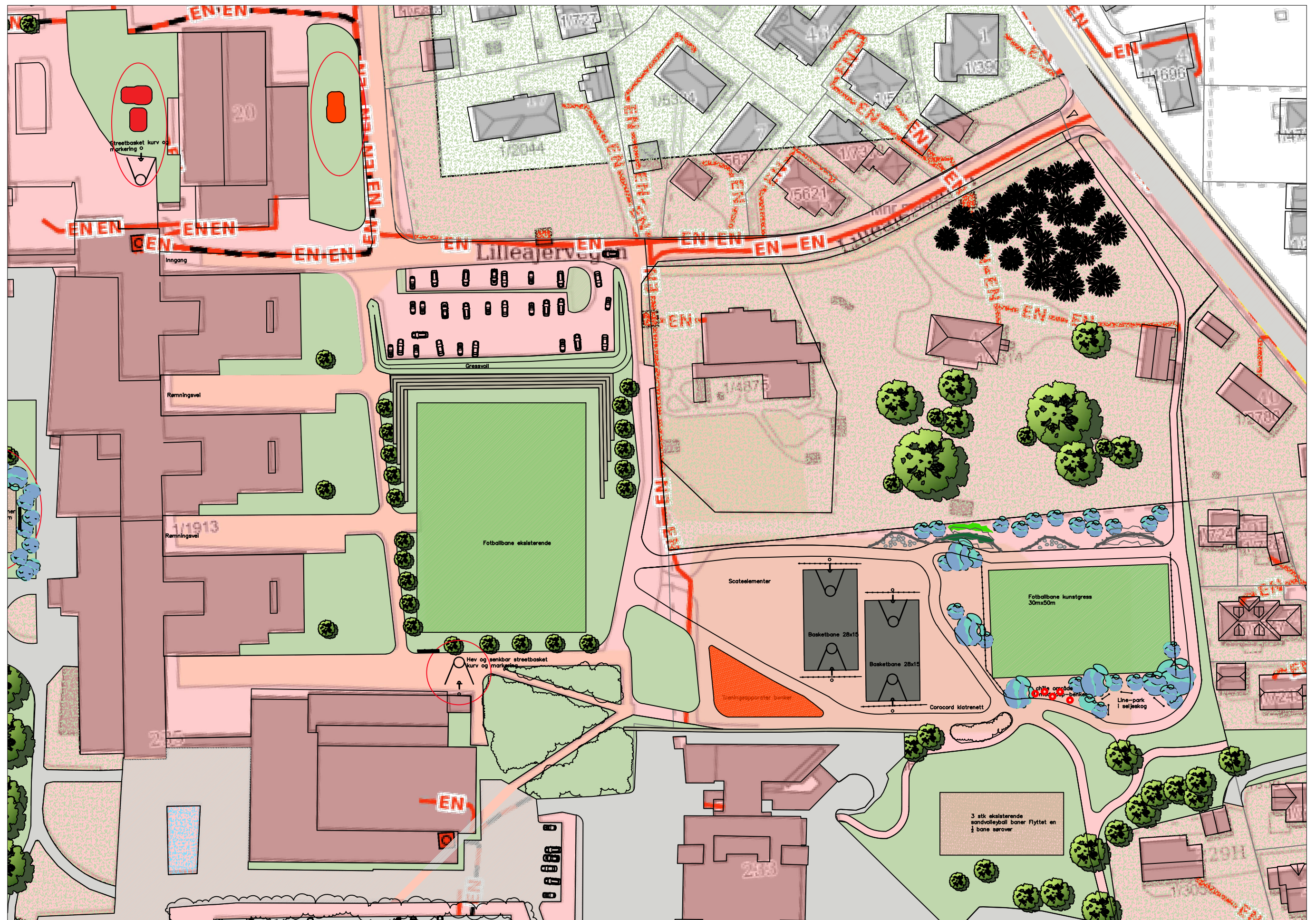
Eidsiva EL— ledningskart, 1:1000 i A3
