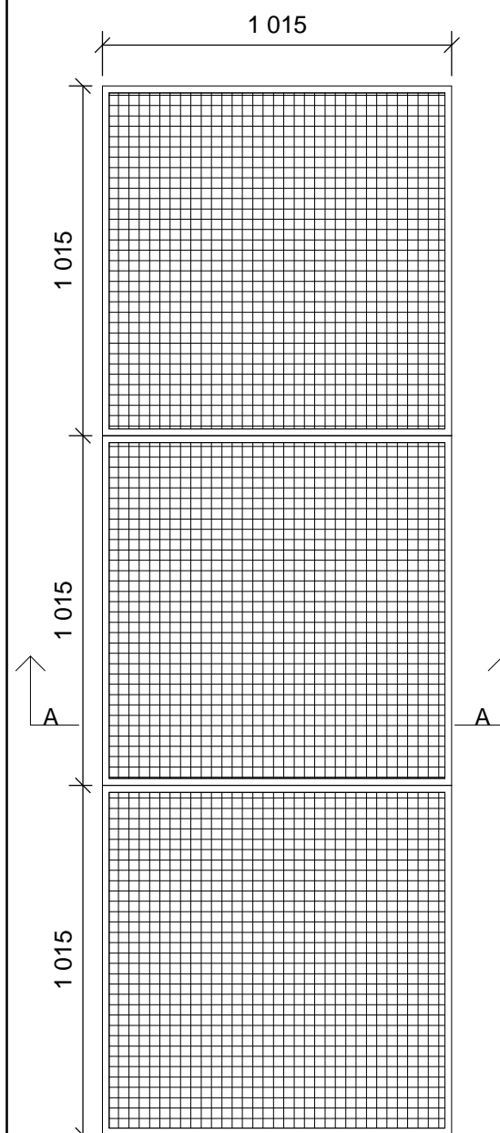
Prefabrikkert granulatopsamlingskum
