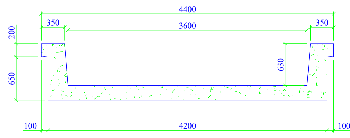
SNITT A-A BRUPLATE 1:30
