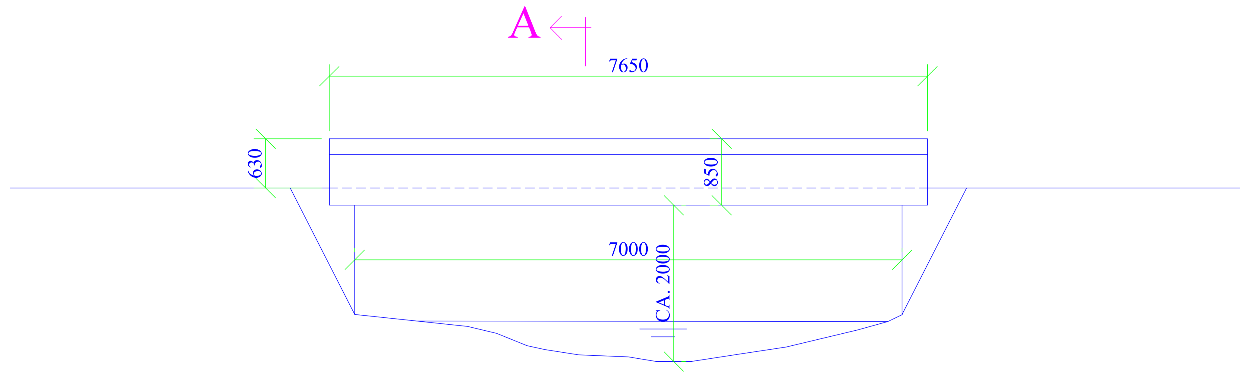
OPPRISS SETT FRA OPPSTRØMS SIDE 1:50
