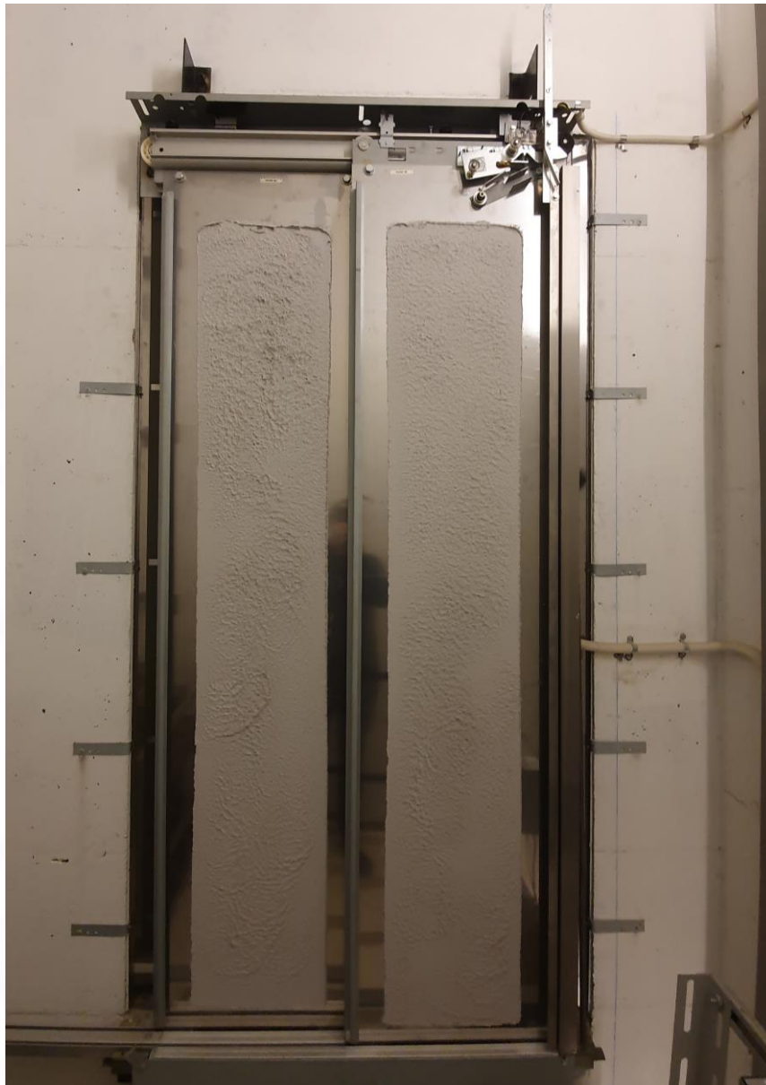
2.01.6 Bilde av sjaktdør på innsiden av sjakten. Innfesting med ekspansjonsbolter.
