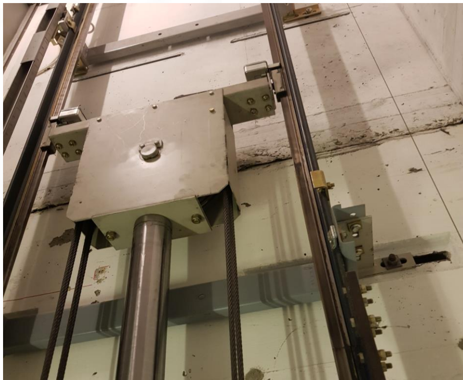
2.01.6 Sjakt – festet med ekspansjonsbolter og ankerskinner.
