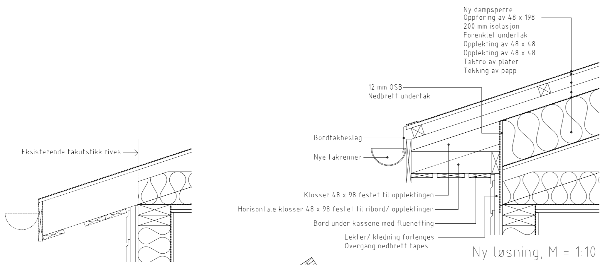
Eks. utstikk, M = 1:10
