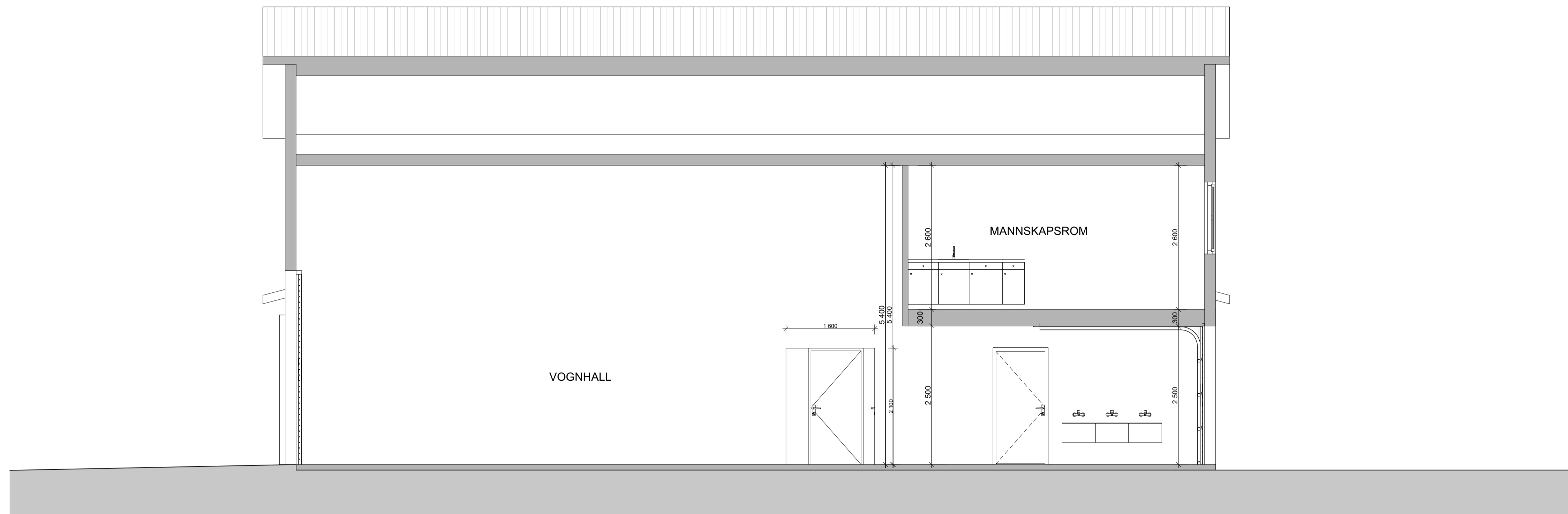
SNITT A-A. EKSISTERENDE
