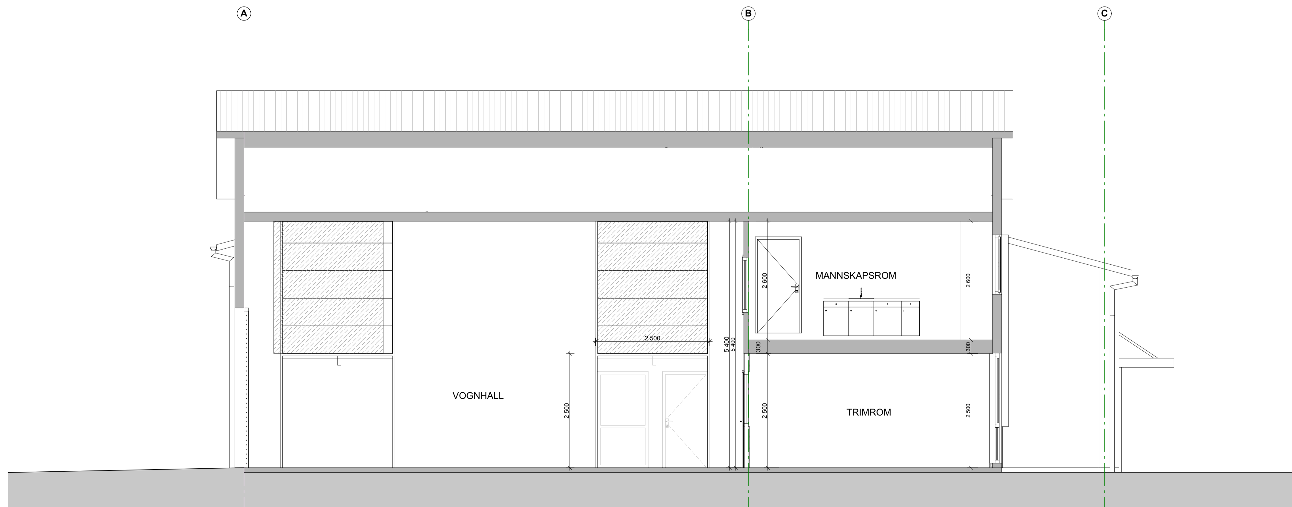
SNITT A-A. PLANLAGT STATUS
