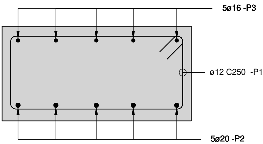
SNITT A-A ARMERING 1:10
