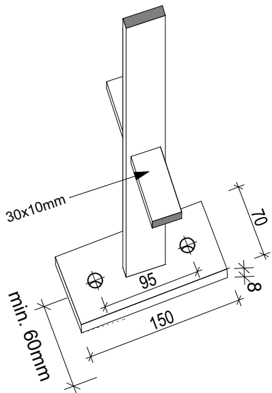
Axonometri, ovenfra
