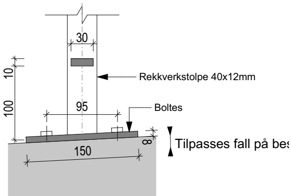
Detalj 02 for innfesting av rekkverk
