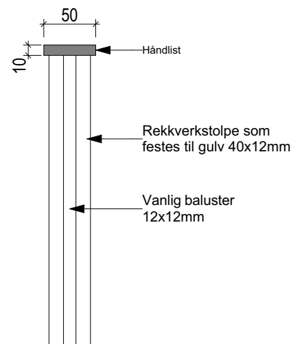
Detalj 01 rekkverk
