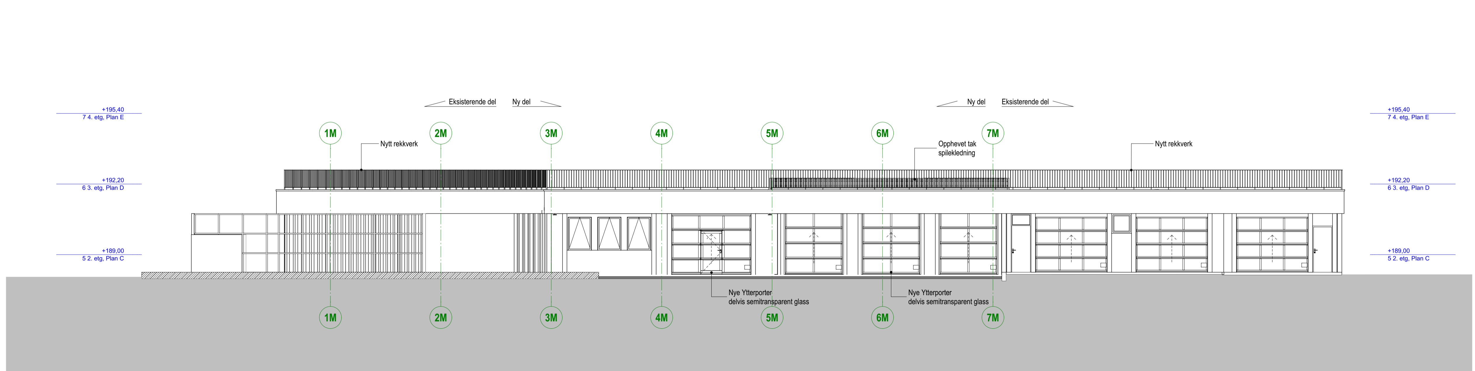
1:100 10M 45.2 Fasade Vest
