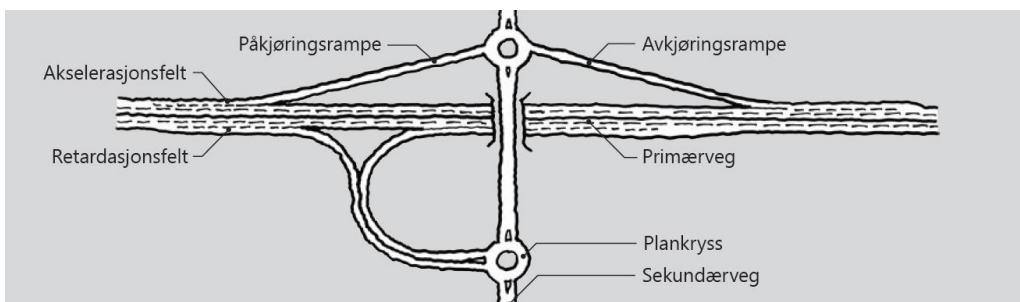
Figur D.17: Planskilt kryss – kryselementer
