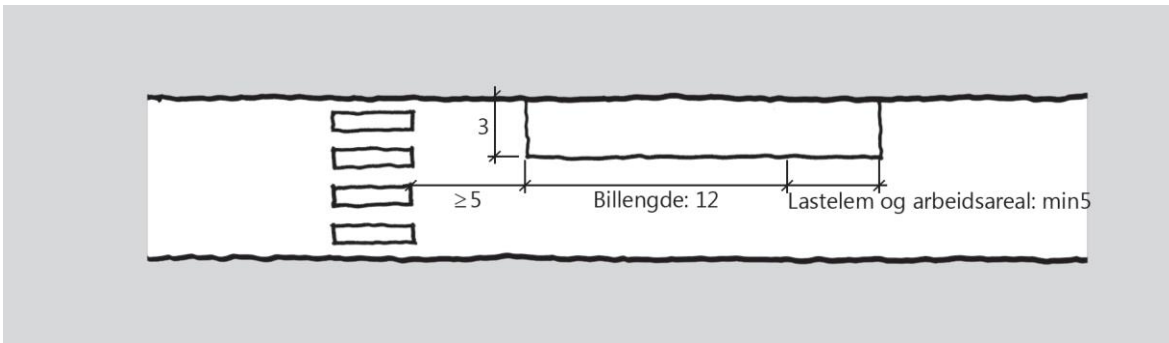
Figur D.51: Varelevering langs kantstein (mål i m)
