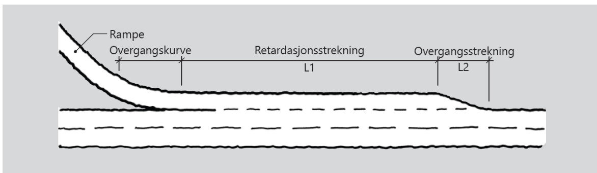
Figur D.19. Standardutforming av parallellført retardasjonsfelt
