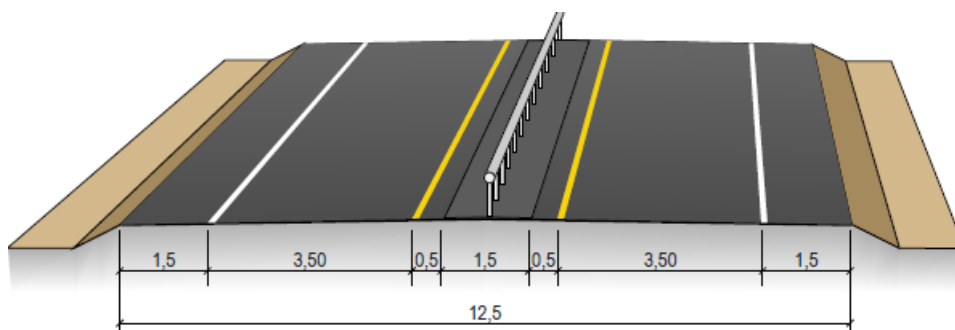
Figur C.2: Tverrprofil for H5, bredde 12,5 (mål i m)
