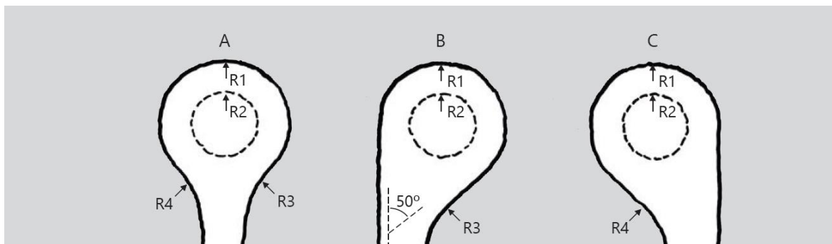
Figur D.48: Utforming av snuplasser
