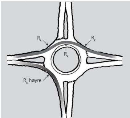
Figur D.11: Prinsipp for avbøyning i en rundkjøring
