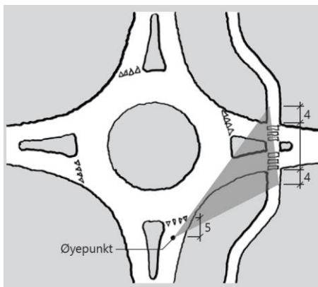
Figur D.16: Sikt til gangfelt (mål i m)
