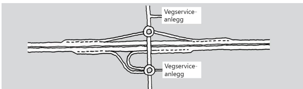
Figur D.46: Eksempel på plassering av serviceanlegg
