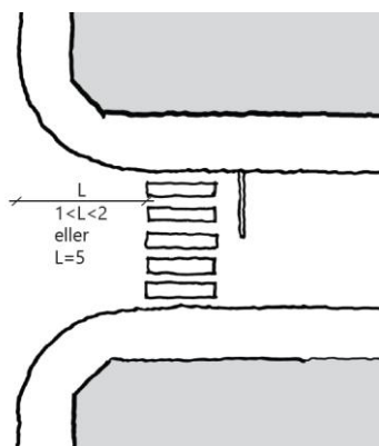
Figur D.33: Plassering av gangfelt i gater
