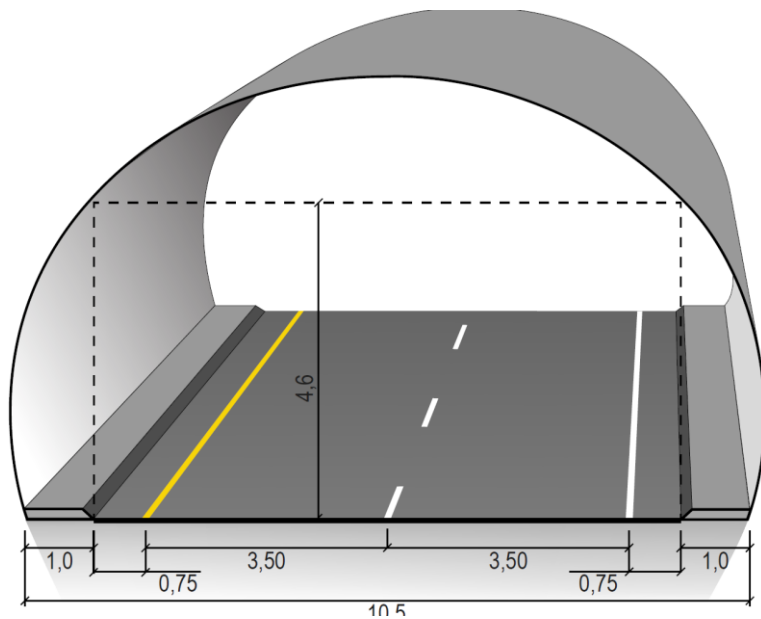
Figur V1.8 Tunnelprofil T10,5 (mål i m)
