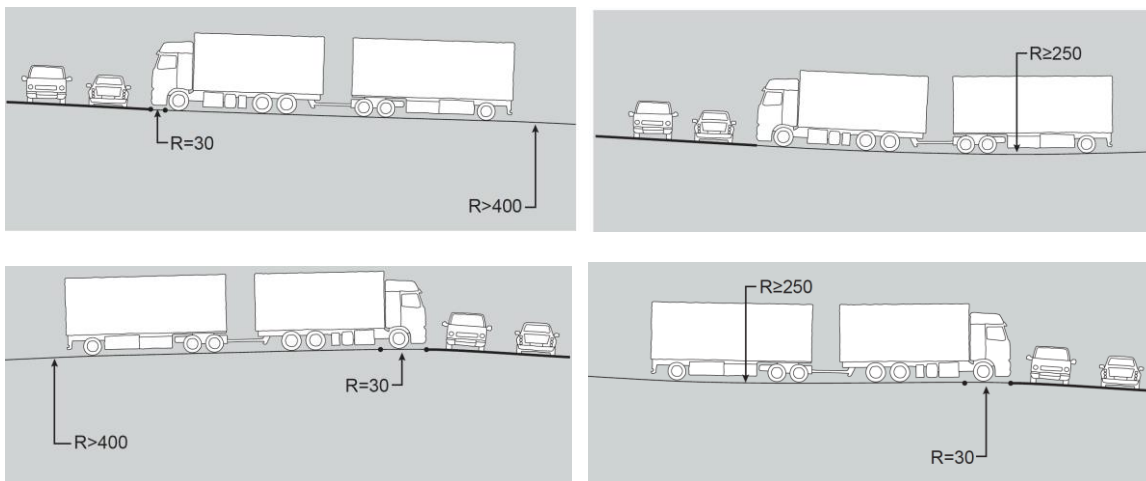
Figur D.2: Krav til sekundærvegens vertikale linjeføring i kryssområdet
