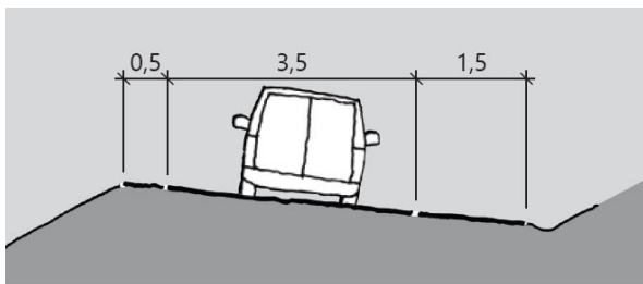
Figur D.18: Rammens tverrprofil (mål i m)
