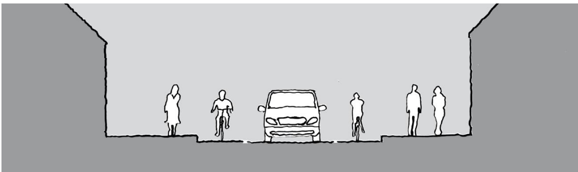
Figur D.32: Envegsregulert gate med sykkelfelt i begge retninger. Minste bredde mellom kantstein bør være 6,5 m
