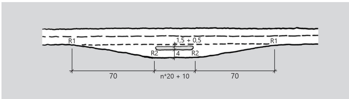
Figur D.37: Busslomme med trafikkdeler, n angir hvor mange busser som forventes å stoppe samtidig (mål i m)
