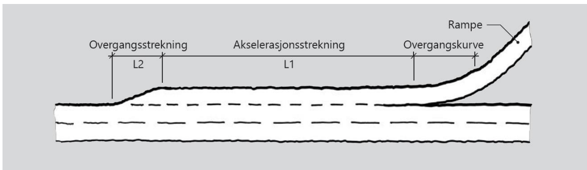
Figur D.20: Standardutforming av parallellført akselerasjonsfelt
