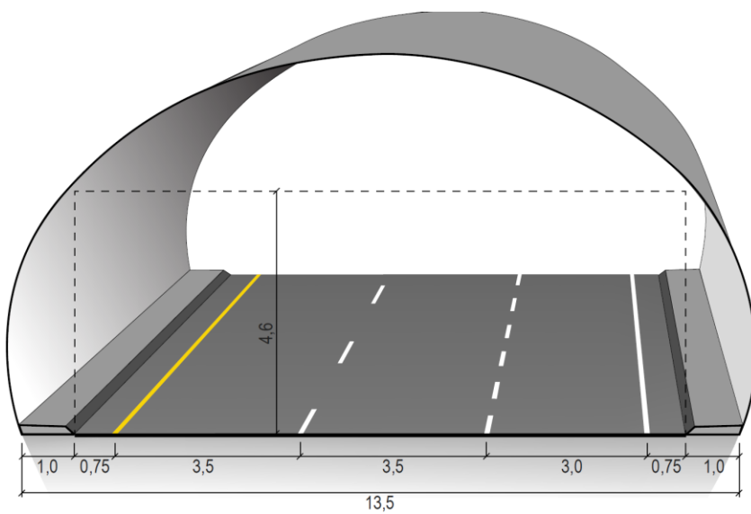
Figur V1.9 Tunnelprofil T13,5 med havarilomme (mål i m)
