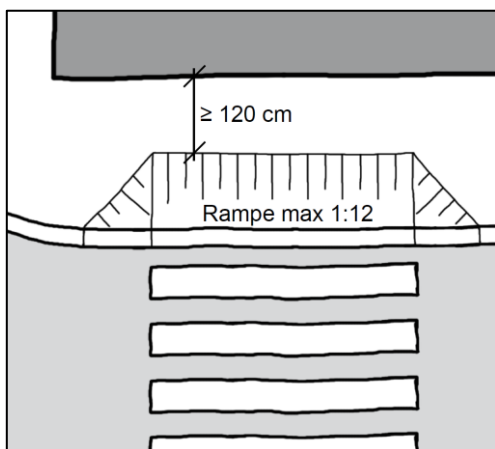
Figur D.39: Nedramping ved gangfelt
