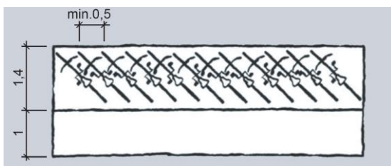
Figur D.45: Sykkelparkering, skråparkering (mål i m)
