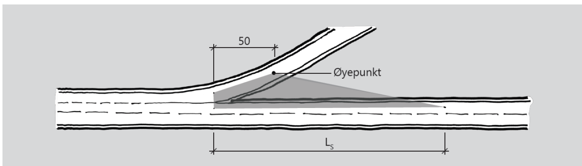
Figur D.21: Sikt fra påkjøringsrampe (mål i m)
