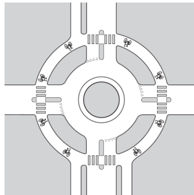
Figur D.13: Prinsipløsning for sykkel i rundkjøring, eksempel 2
