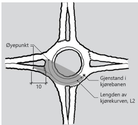
Figur D.15: Sikt fremover i rundkjøringen (mål i m)
