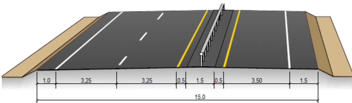
Figur C.3: Tverrprofil H5 med forbikjøringsfelt, bredde 15 (mål i m)
