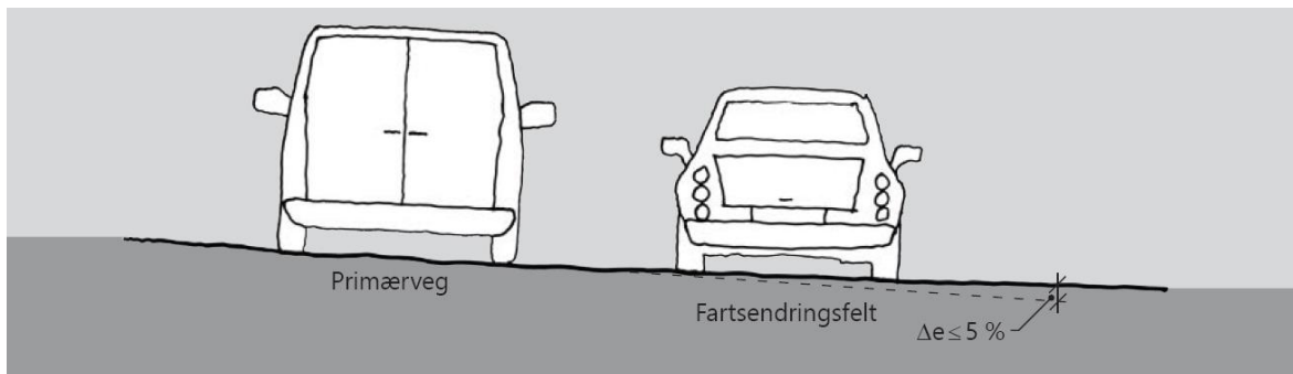
Figur D.22: Forskjell i tverrfall mellom primærveg og fartsendringsfelt
