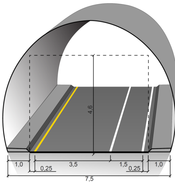
Figur V1.18 Tunnelprofil T7,5 (mål i m). Brukes for av- og påkjøringsramper med ett kjørefelt der havarett kjøretøy kan passeres.
