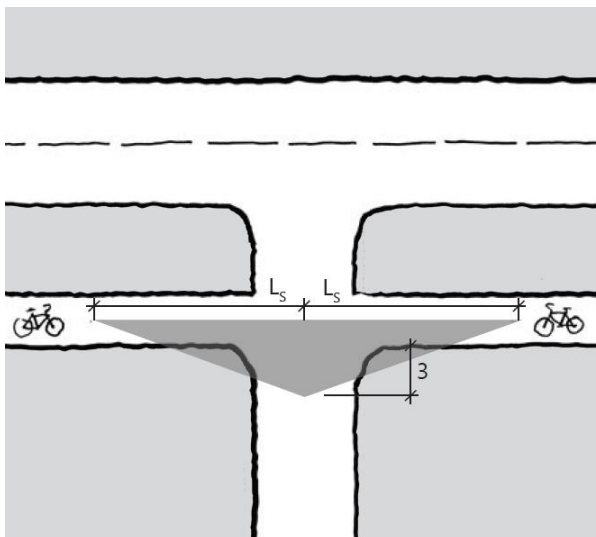
Figur D.29: Sikt mellom gang- og sykkelveg/sykkelveg og avkjørsel (mål i m)
