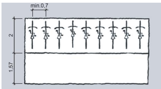
Figur D.44: Sykkelparkering, vinkelrett parkering (mål i m)
