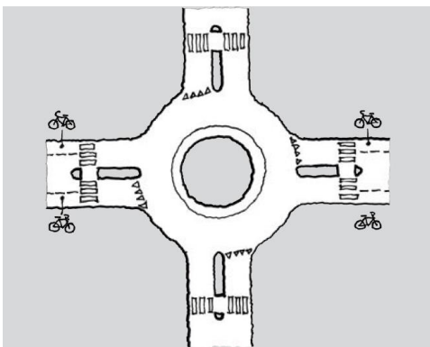
Figur D.12: Prinsipløsning for sykkel i rundkjøring, eksempel 1
