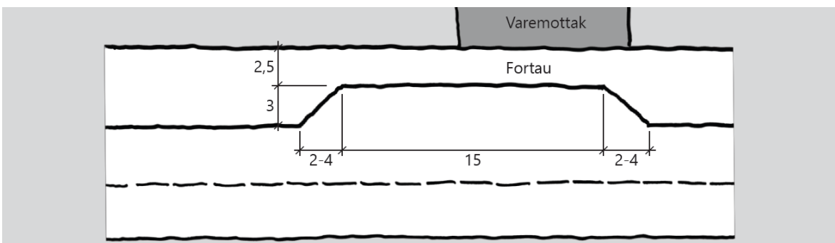
Figur D.52: Varelevering i lomme (mål i m)
