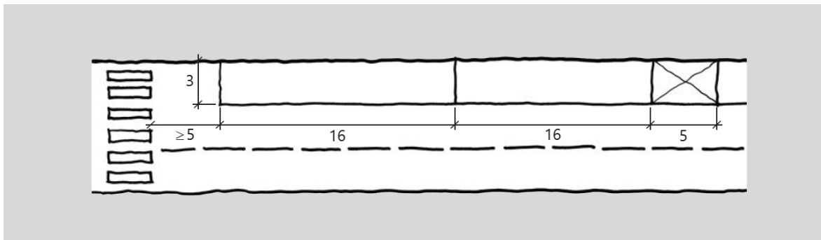
Figur D.43: Kantparkering for buss (mål i m)
