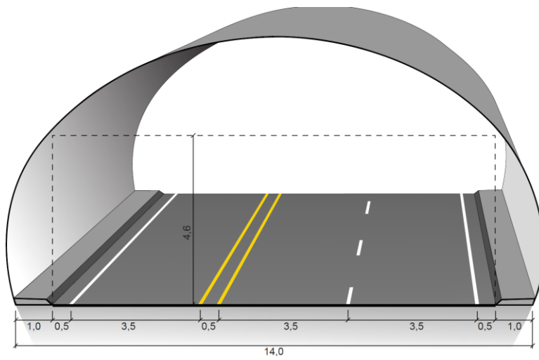
Figur V1.7 Tunnelprofil T14 med forsterket midtoppmerking og forbikjøringsfelt (mål i m)
