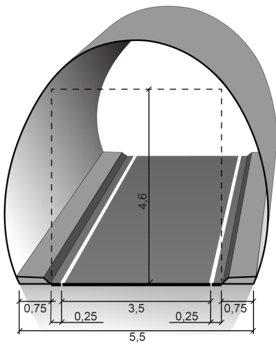
Figur V1.19 Tunnelprofil T5,5 (mål i m). T5,5 brukes for rømningstunnel
