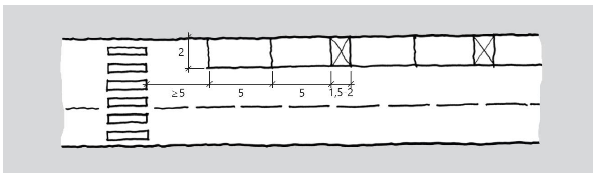
Figur D.40: Langsgående parkering (mål i m)
