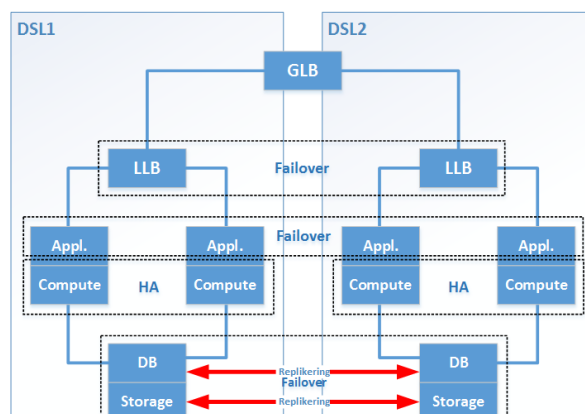
Figur 5 Tradisjonell applikasjonsarkitektur
