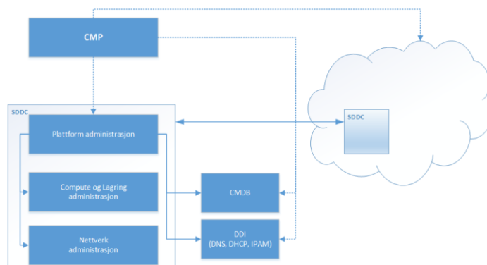
Figur 20 Generisk provisjoneringsverktøy
