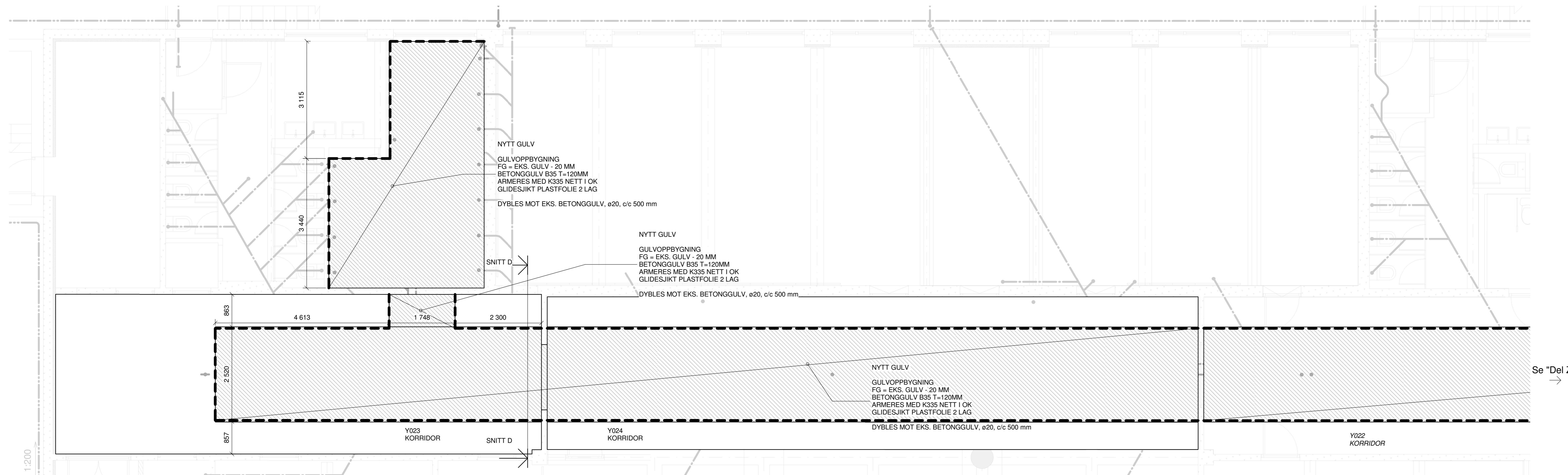
GULVSTØPEPLAN KJELLER - DEL Y 1 : 50
