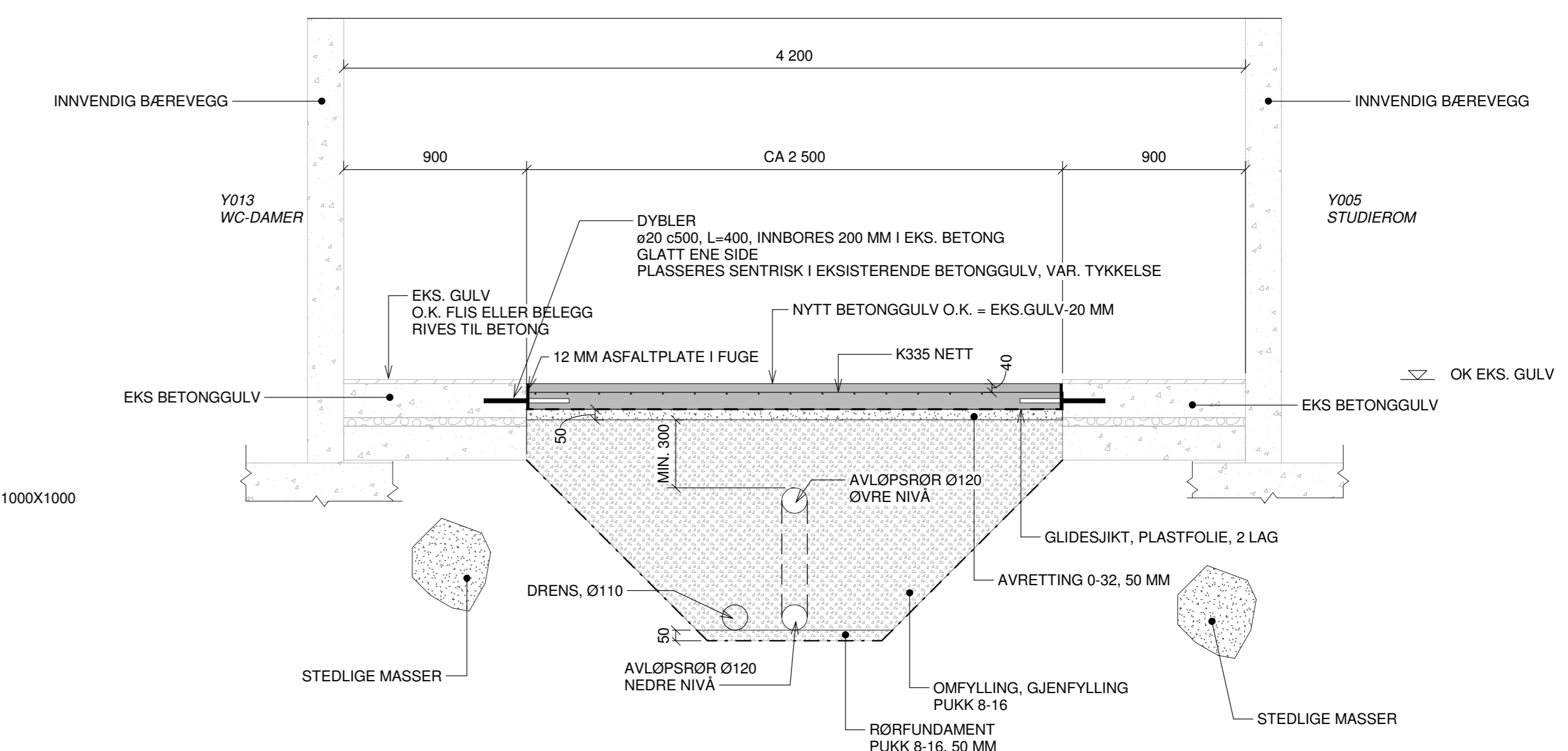
SNITT D-D - GRØFT MED NYTT BETONGGULV, TYP. OPPBYGGING 1 : 20
