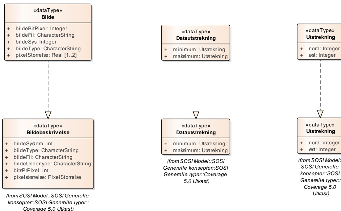
Figur 4: Realisering av datatyper
