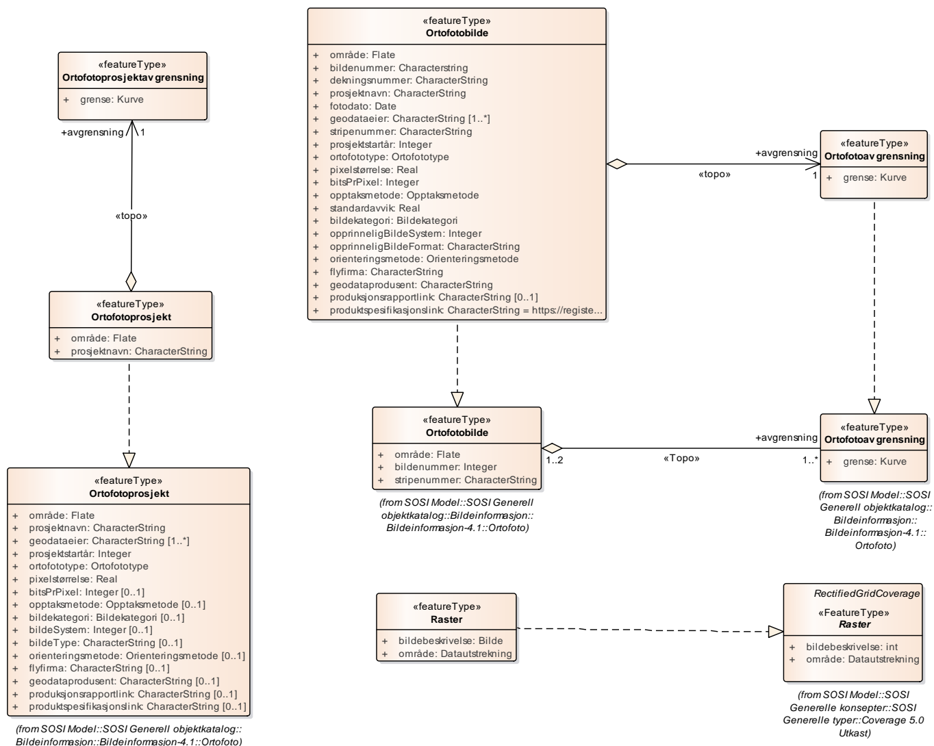
Figur 3: Realisering av objekttyper
