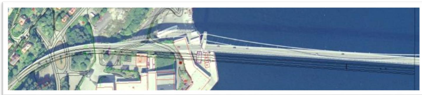
Figur B.7: Eksempler som viser at terrenngmodellen ikke er justert ved tekniske anlegg (bru). Broen tilfredsstillers ikke ortofoto kravet til nøyaktighet i grunnriss. De svarte strekene viser broens virkelige plassering.
