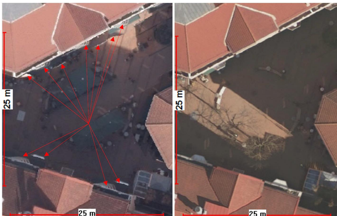
Figur B.10: Venstre bilde viser et eksempel på et sant ortofoto hvor takrenner og andre bygningsdeler vises liggende på bakken. Til høyre er feilen rettet opp i henhold til forventningene til produktet. Eksemplet er laget av Oslo Kommune.
