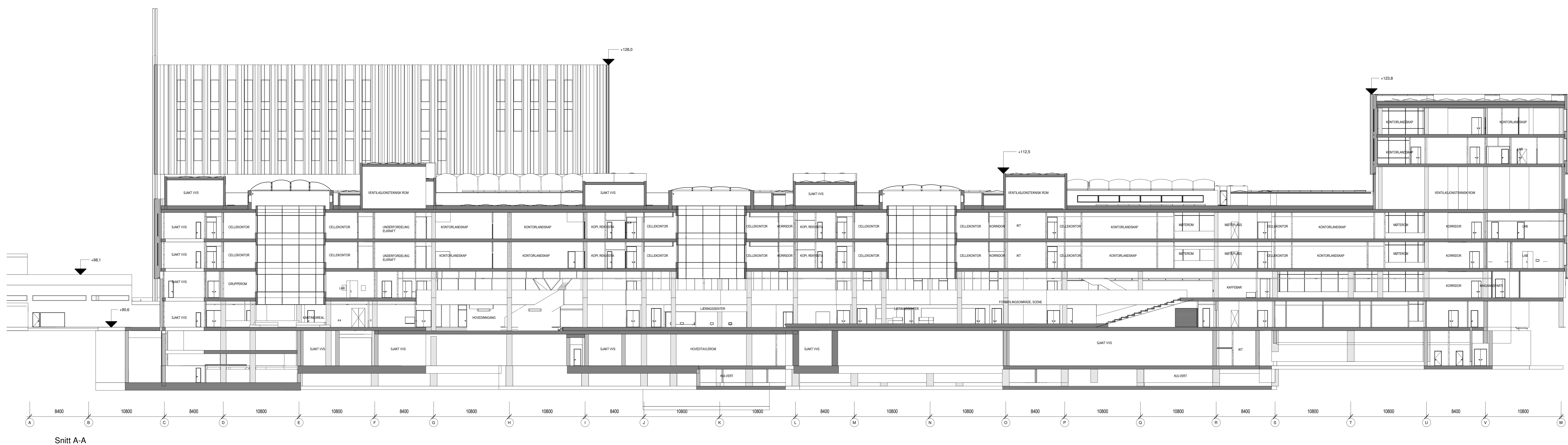
Snitt A-A
