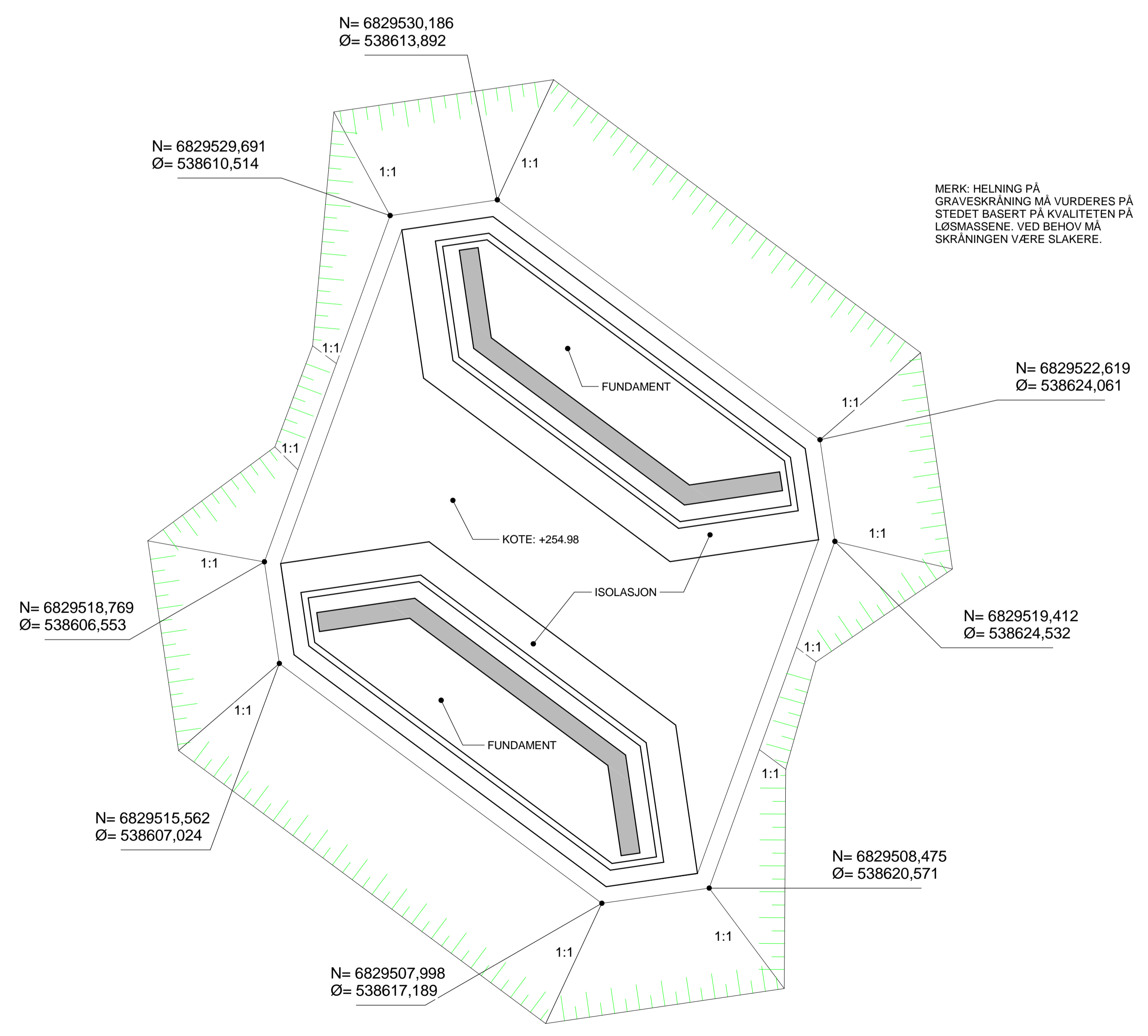
GRAVEPLAN - BRU GIVRAVEGEN 1 : 100
