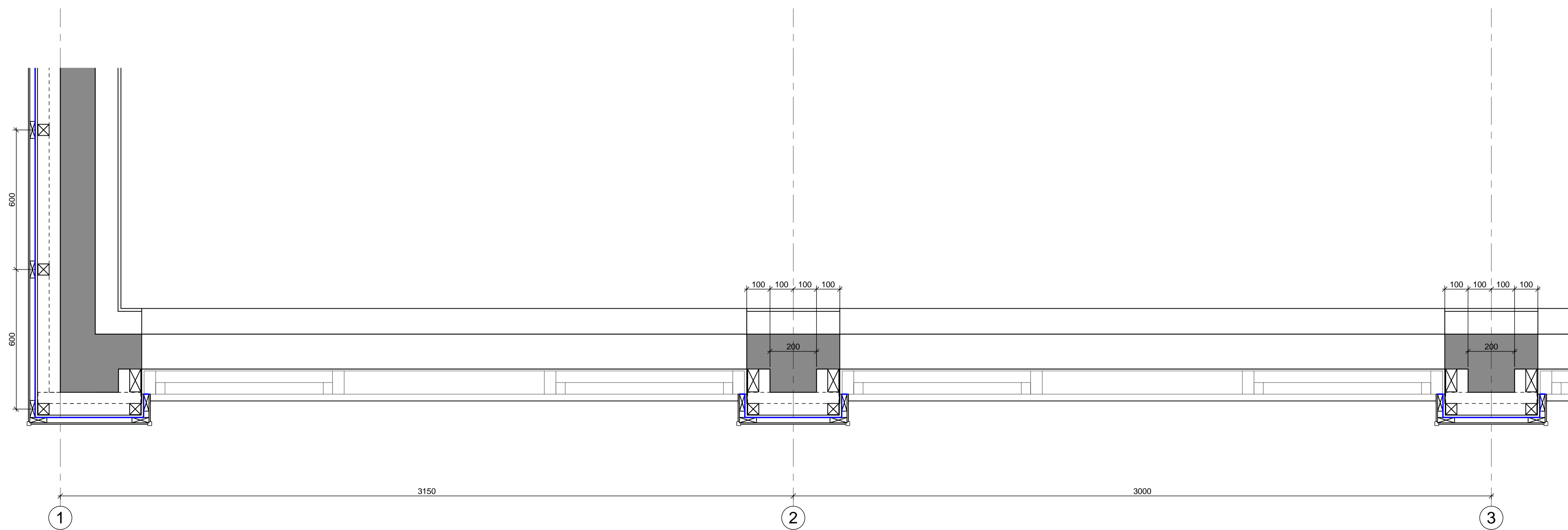
3.etg. skifte vinduer 1:10
