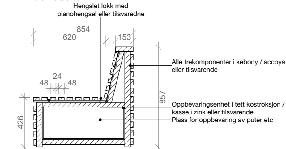
SNITT A-A 1:20
