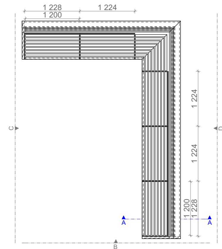
PLAN 1:50
