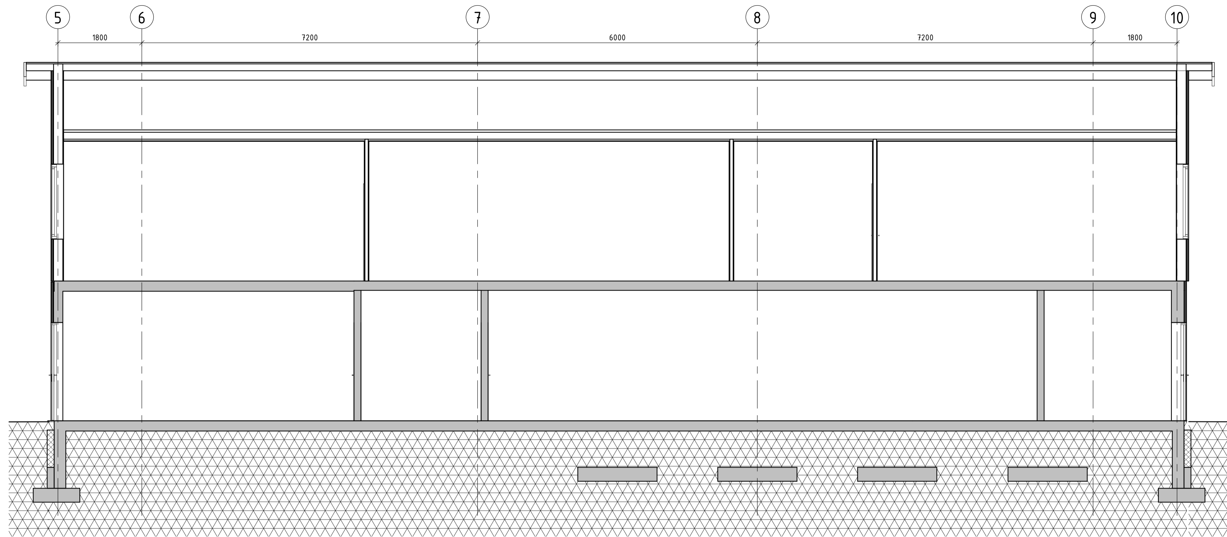
d2 - Snitt akse J bygg D 1 : 50
