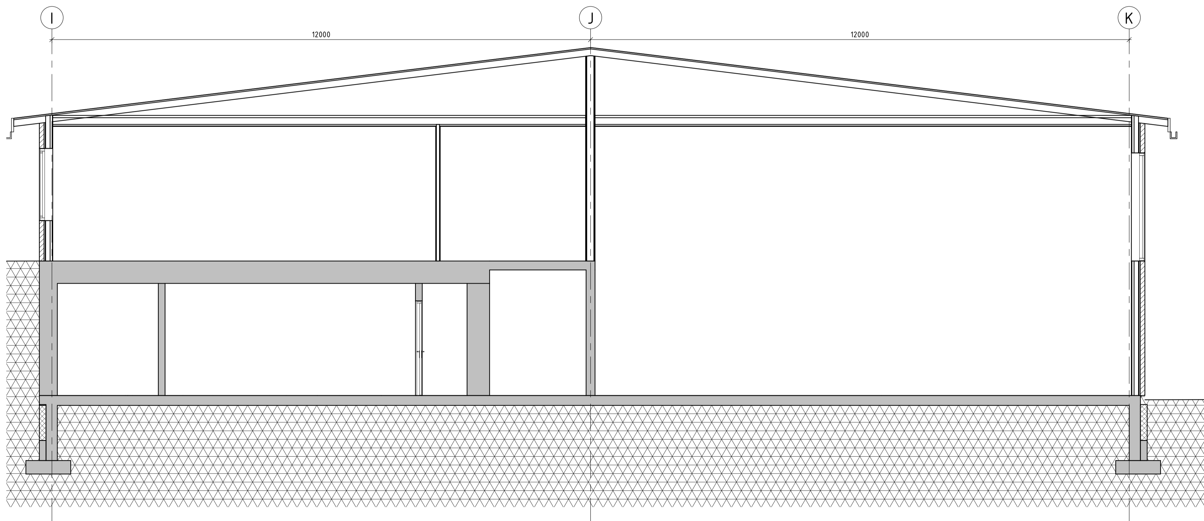
d1 - Snitt akse 7 bygg D1 1 : 50
