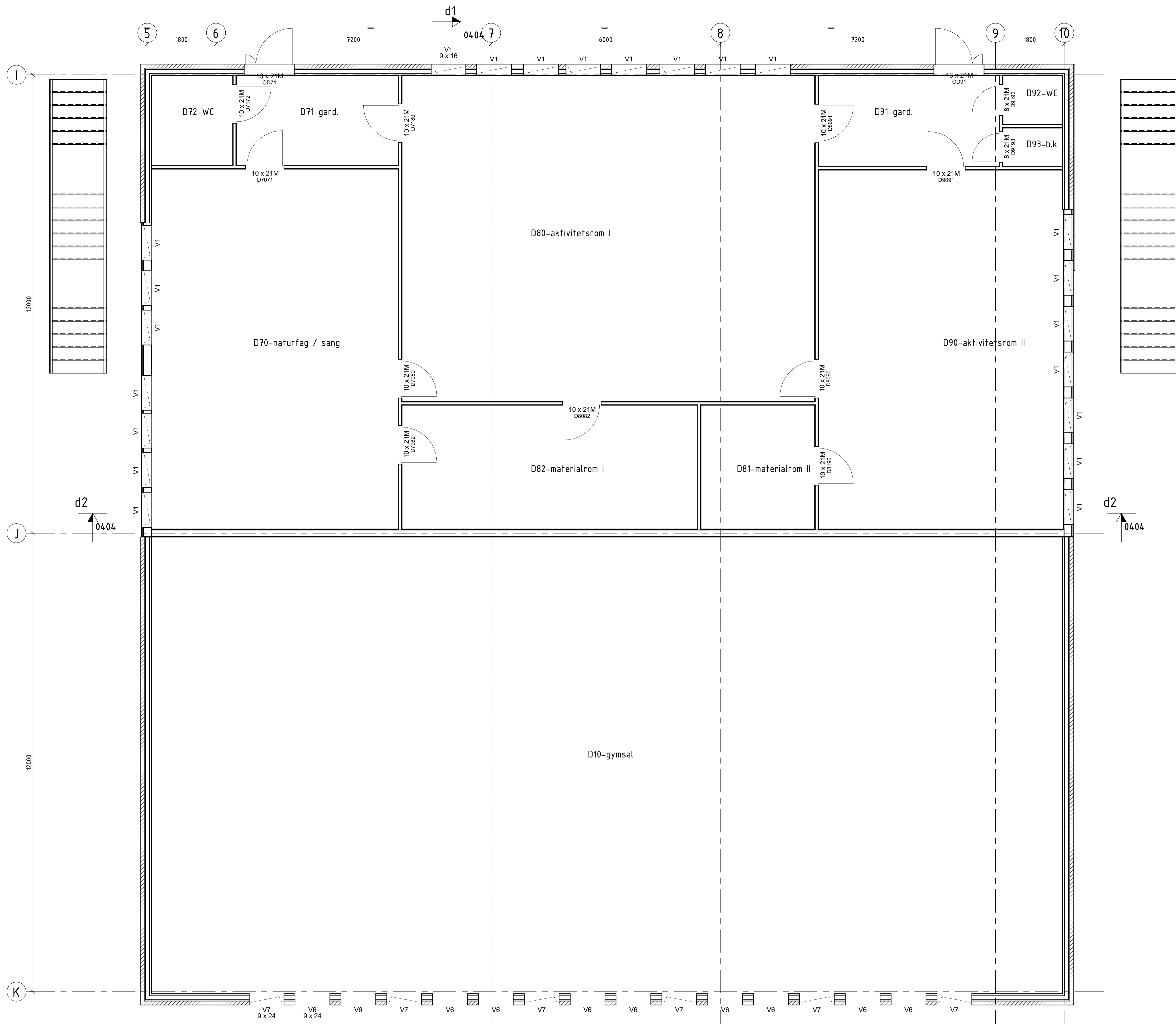
Plan OK+61.2m Bygg D - 1.etg 1 : 50
