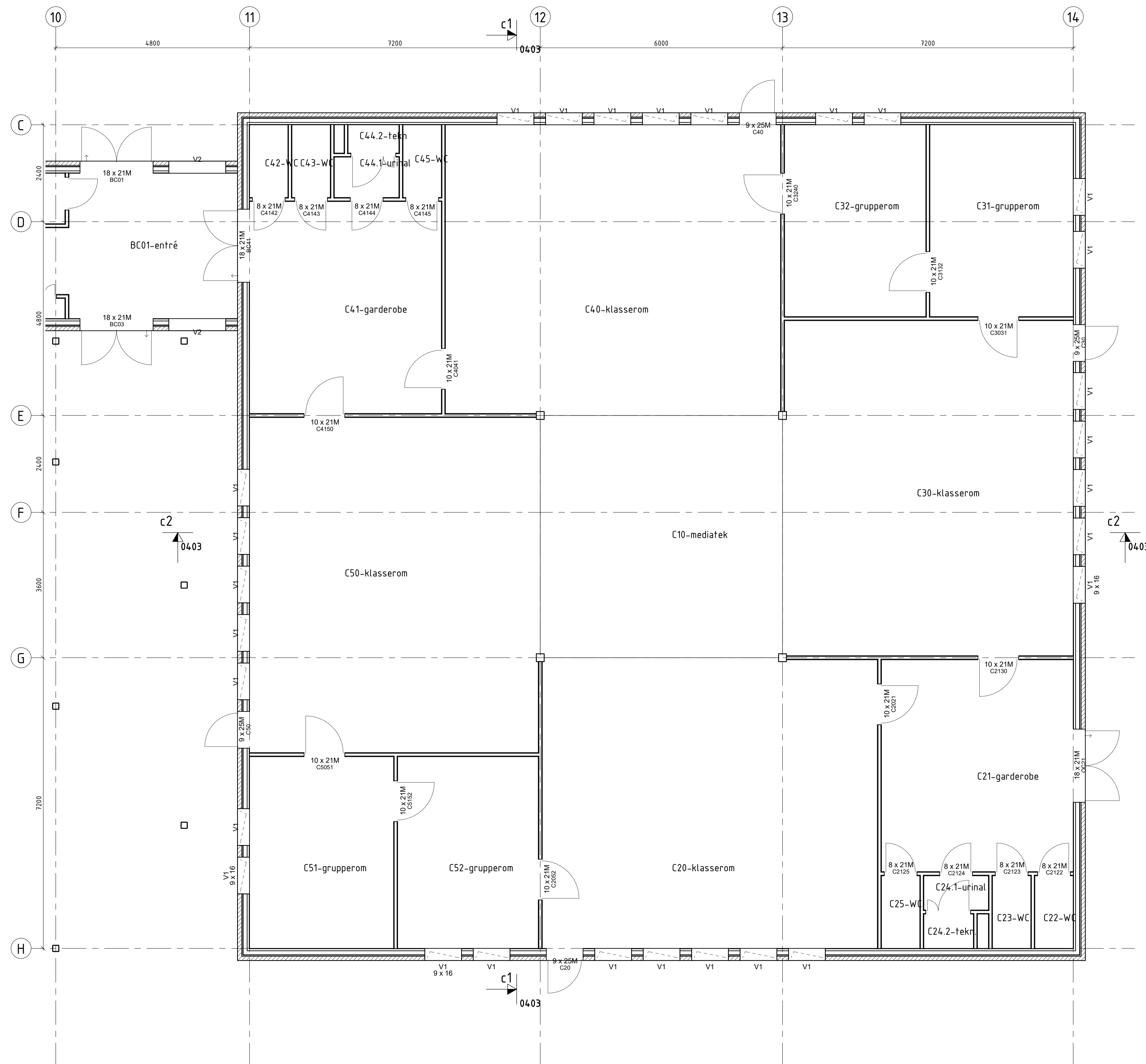
Plan OK+61.2m Bygg C 1: 50
