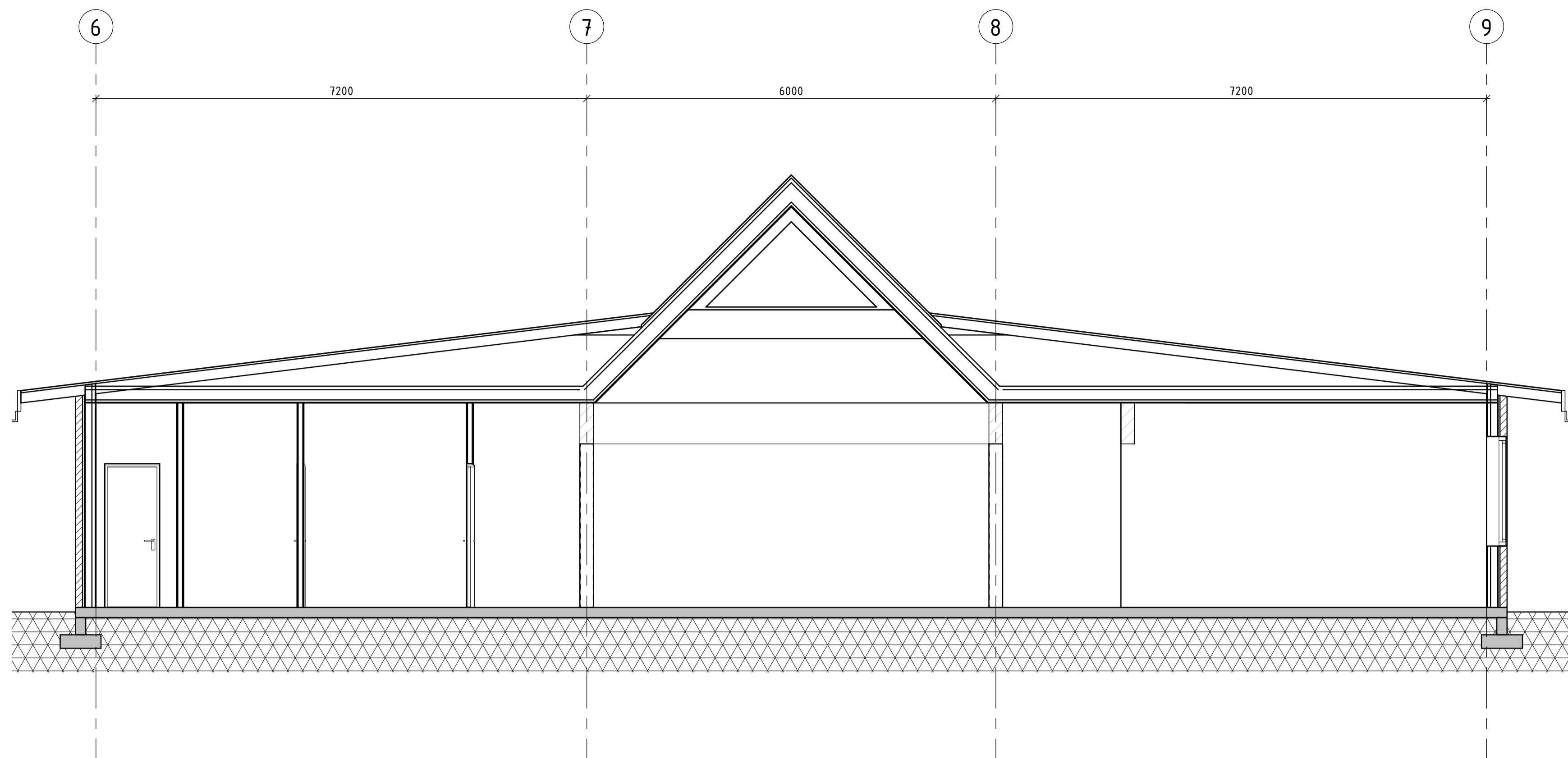
b2 - Snitt akse C bygg B1 1 : 50
