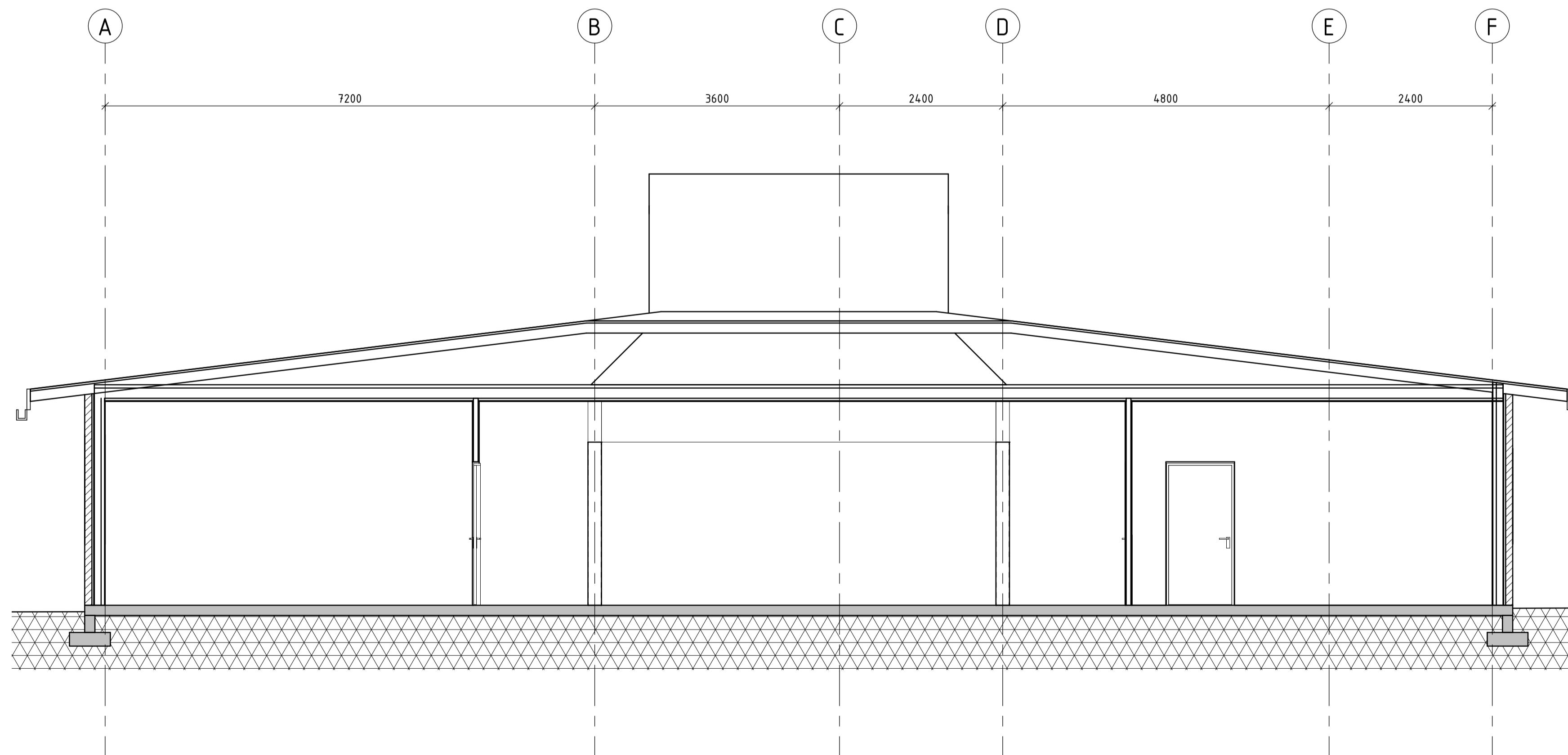
b1 - Snitt akse 7 bygg B2 1 : 50
