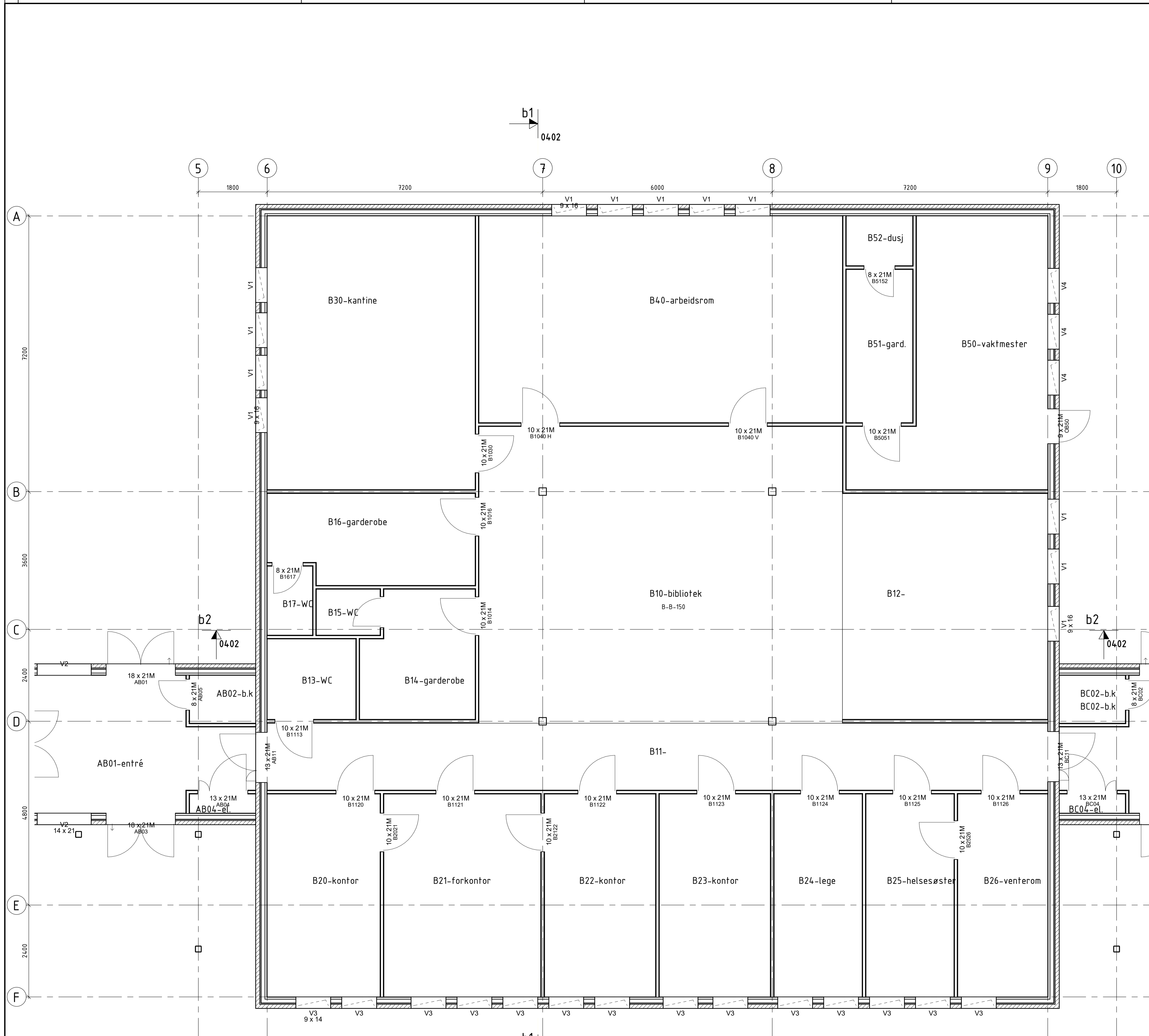
Plan OK+61.2m Bygg B 1 : 50
