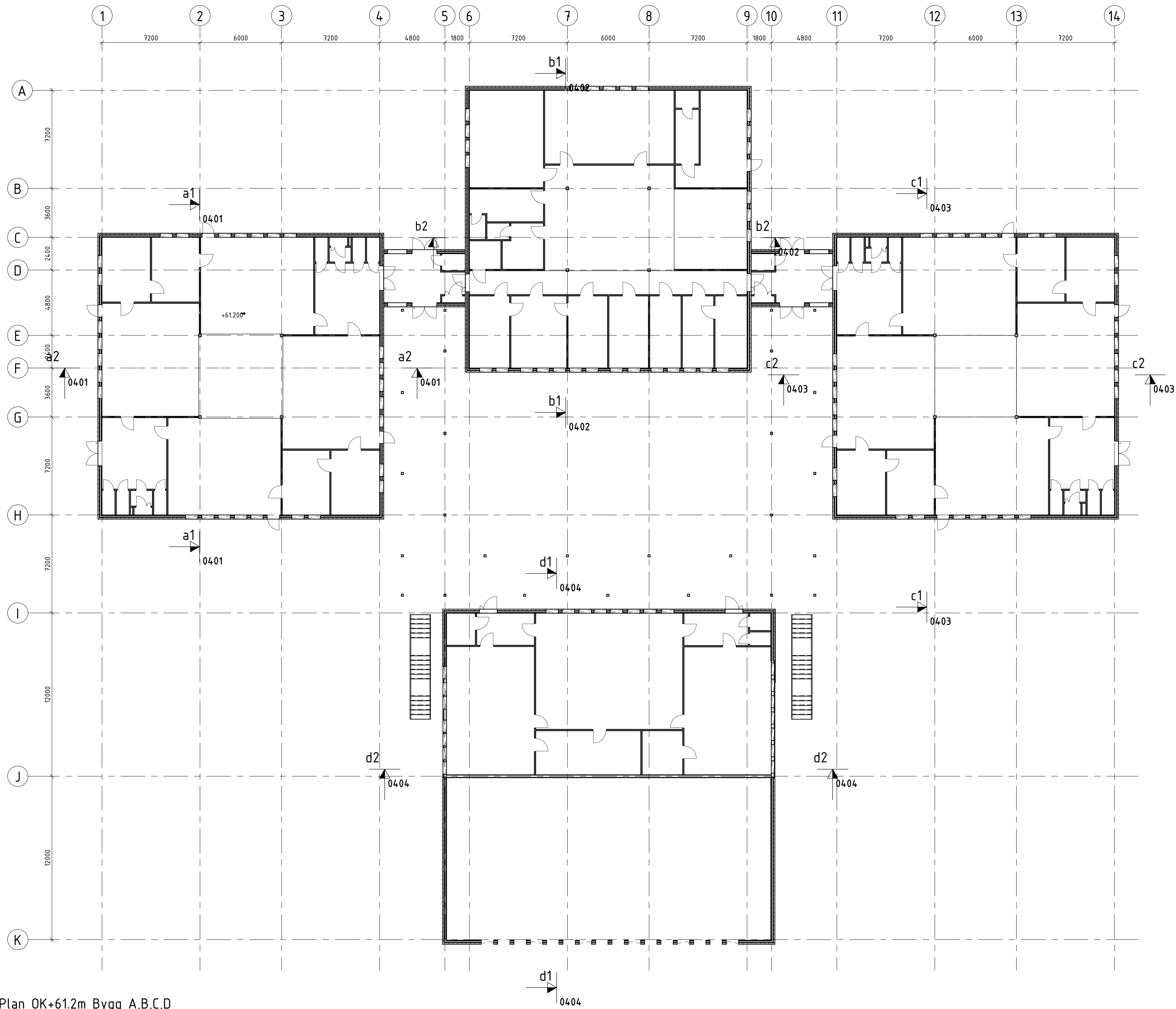
Plan OK+61.2m Bygg A,B,C,D 1 : 150
