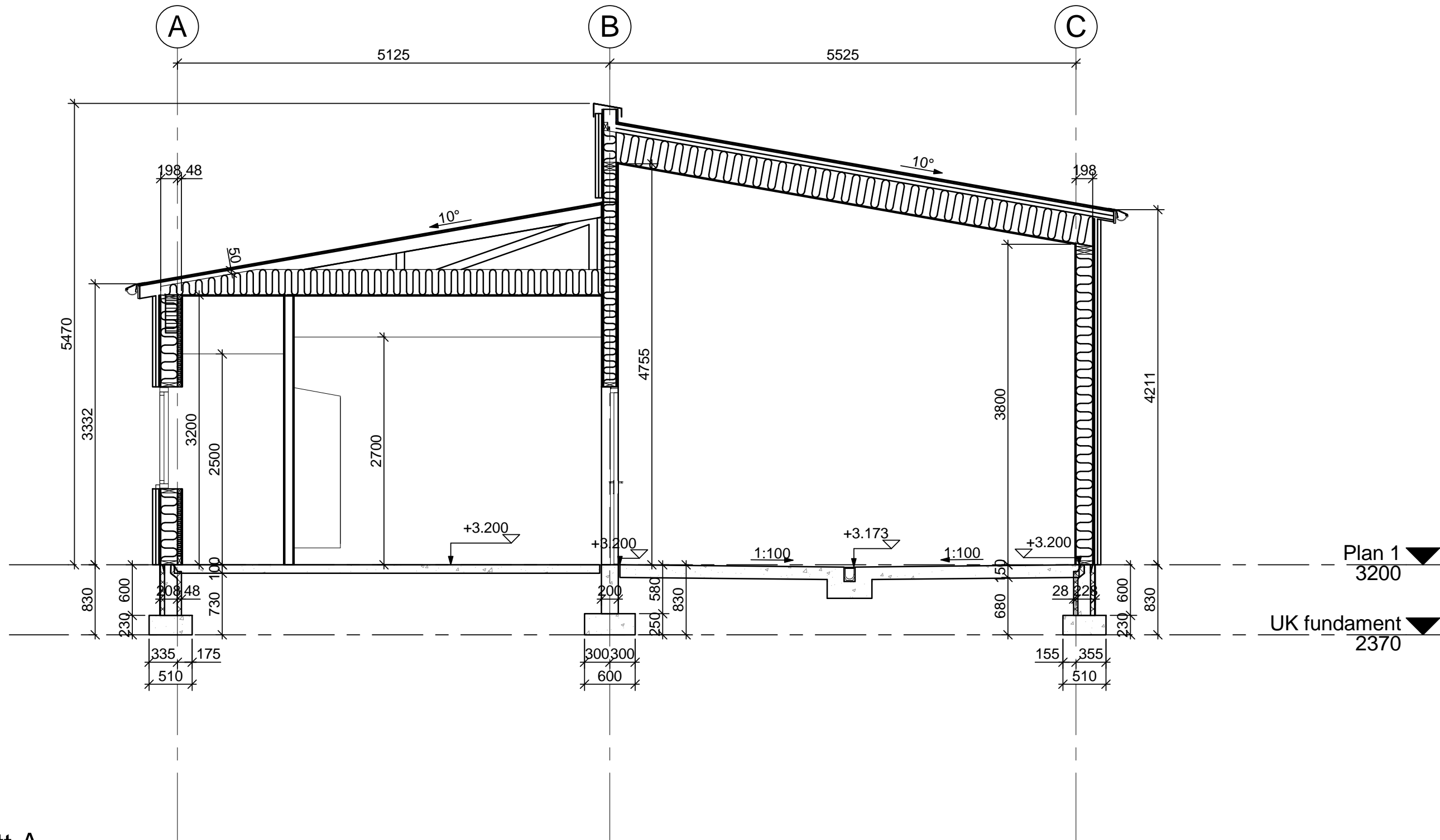
Snitt A 1 : 50
