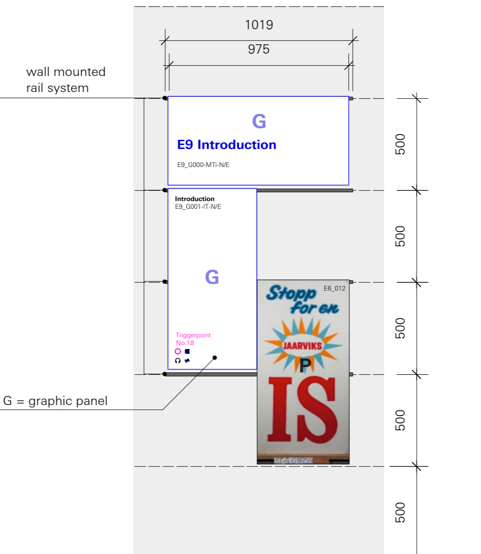
ELEVATION MODULE E9 M 1:20
