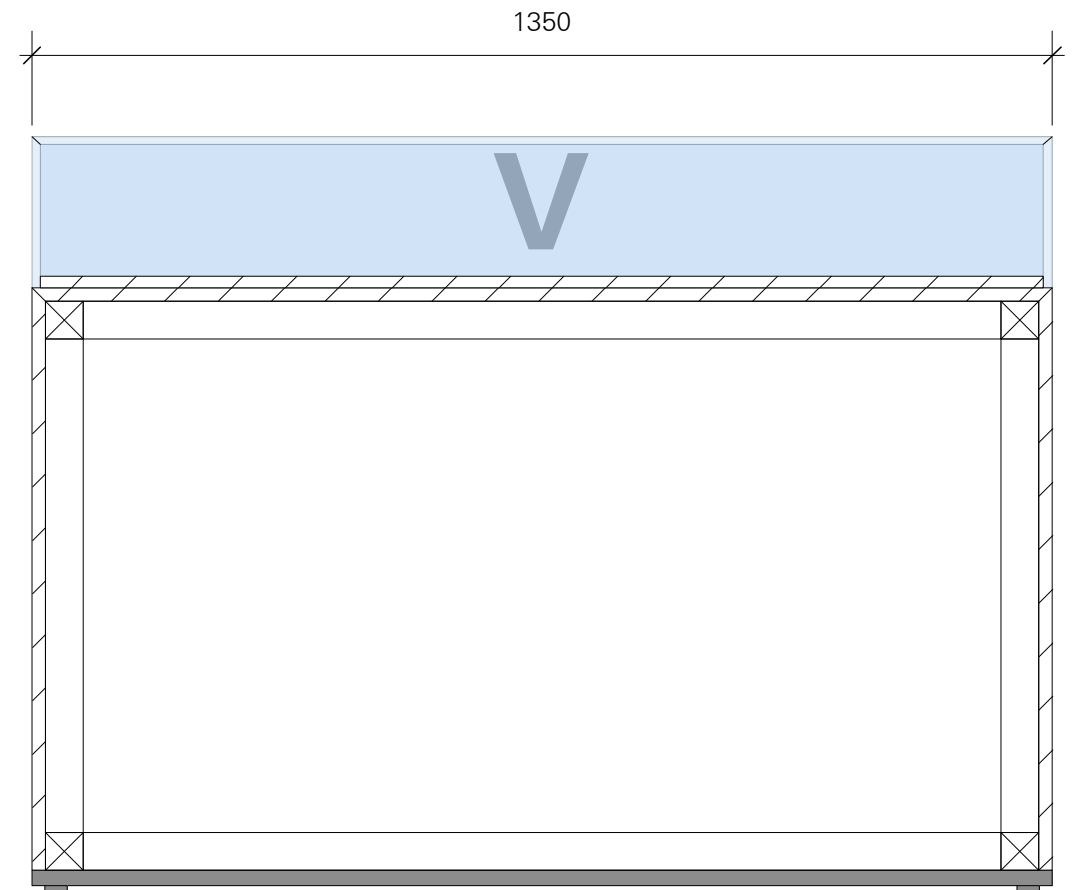
SECTION SHOWCASE MODULE E5, E7 M 1:10
