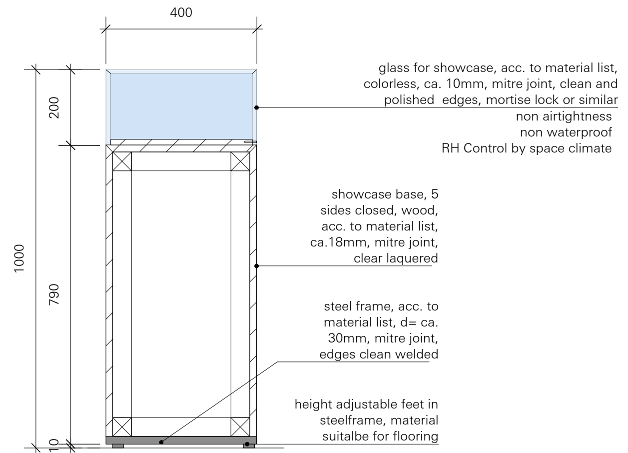
SECTION SHOWCASE MODULE E5, E7 M 1:10
