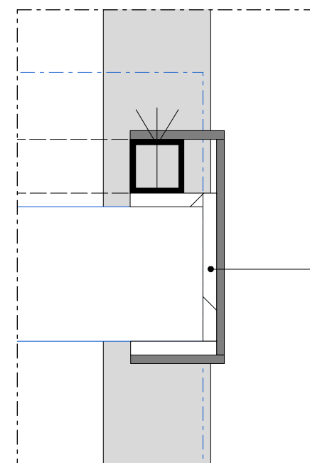
DETAIL 1 MODULE B3b / C7 M 1:2
