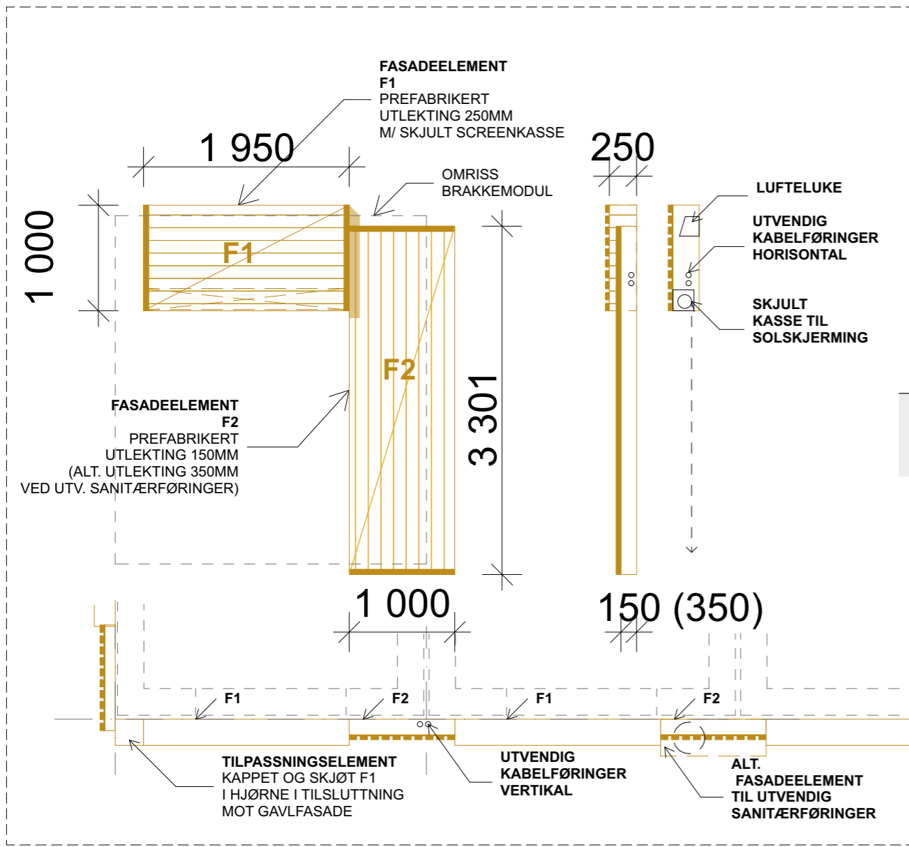
FASADEELEMENT M1:50
