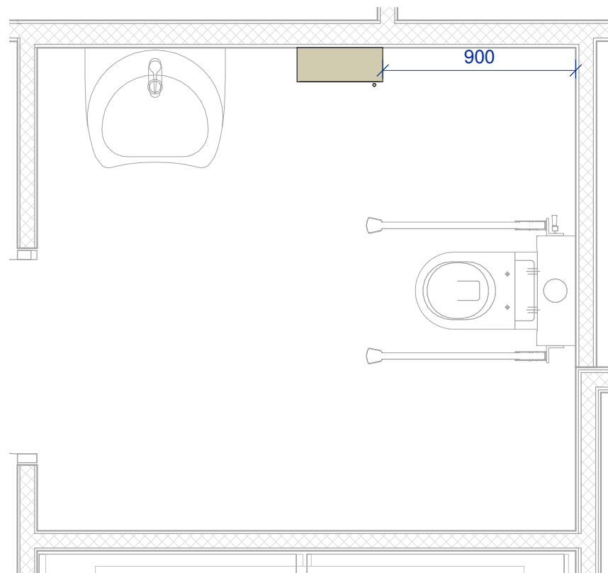
Planutsnitt toalett 1 : 25
