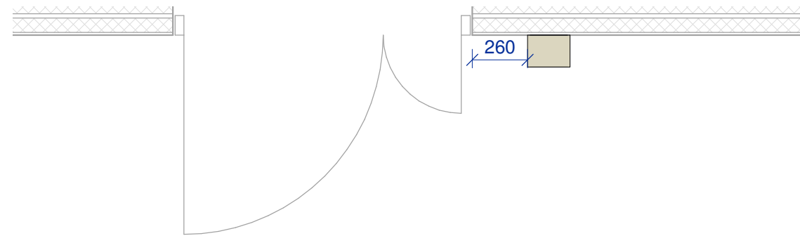
Planutsnitt korridor 1 : 25
