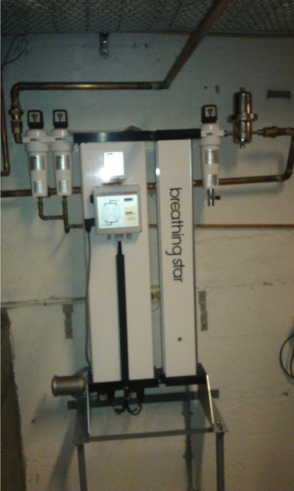
Bilde av eksisterende kombinerte filter- og tørkearrangement 2
