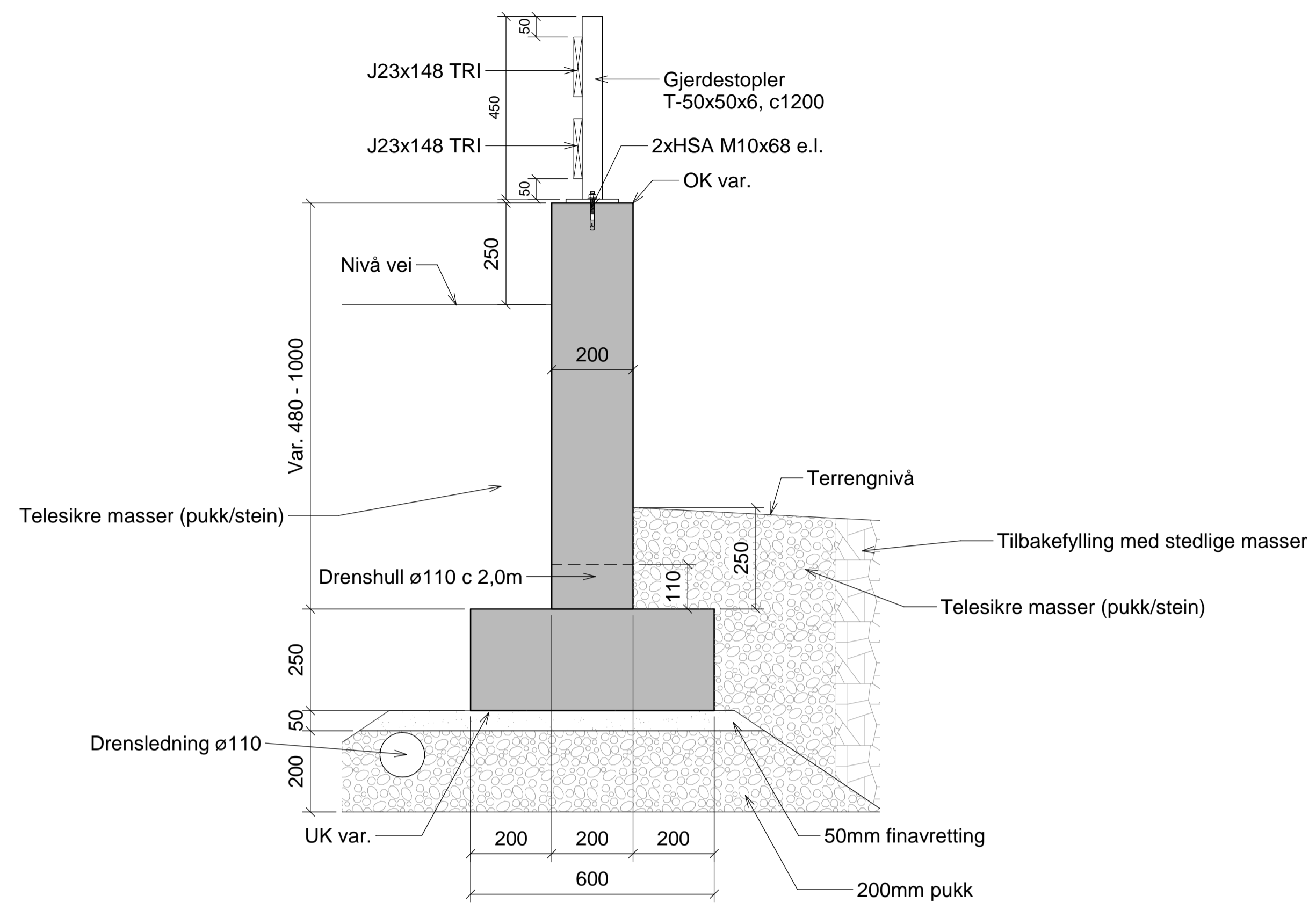
Typisk snitt støttemur 1 : 10
