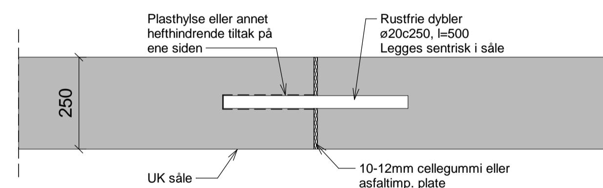
Detalj vertikal fuge støttemur. Horisontalt snitt gjennom bevegesfuge 1:10
