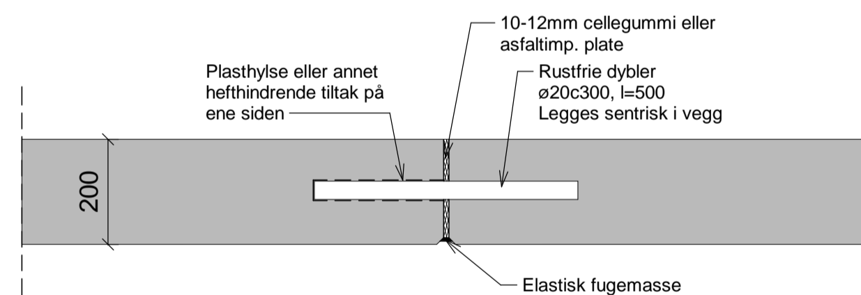
Detalj vertikal fuge støttemur. Horisontalt snitt gjennom bevegesfuge 1:10
