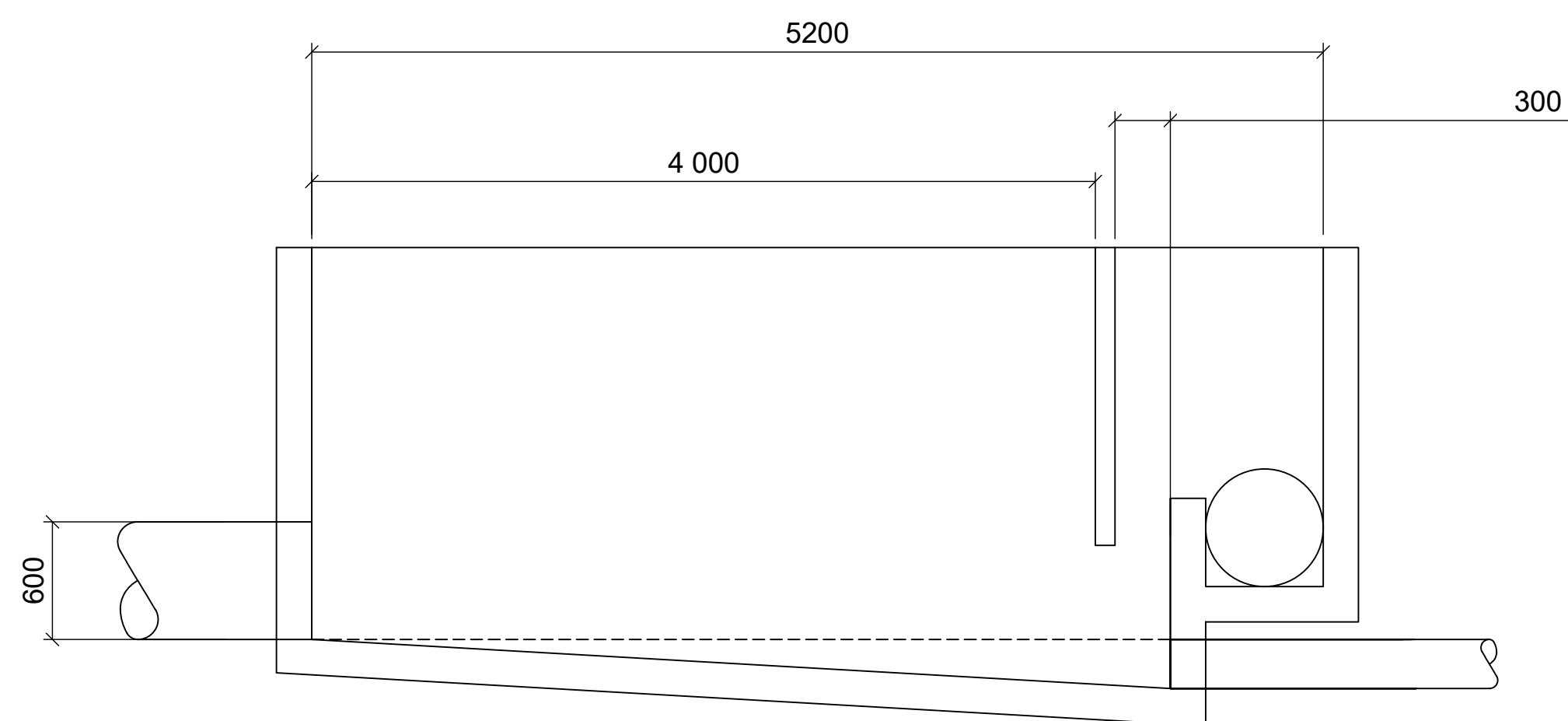
Tverroverløp snitt A-A:
