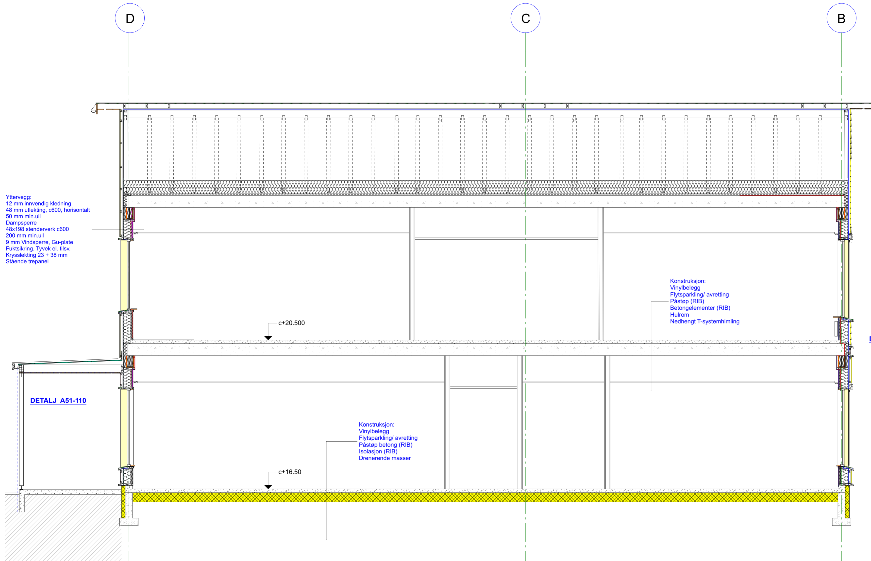
Snitt A
