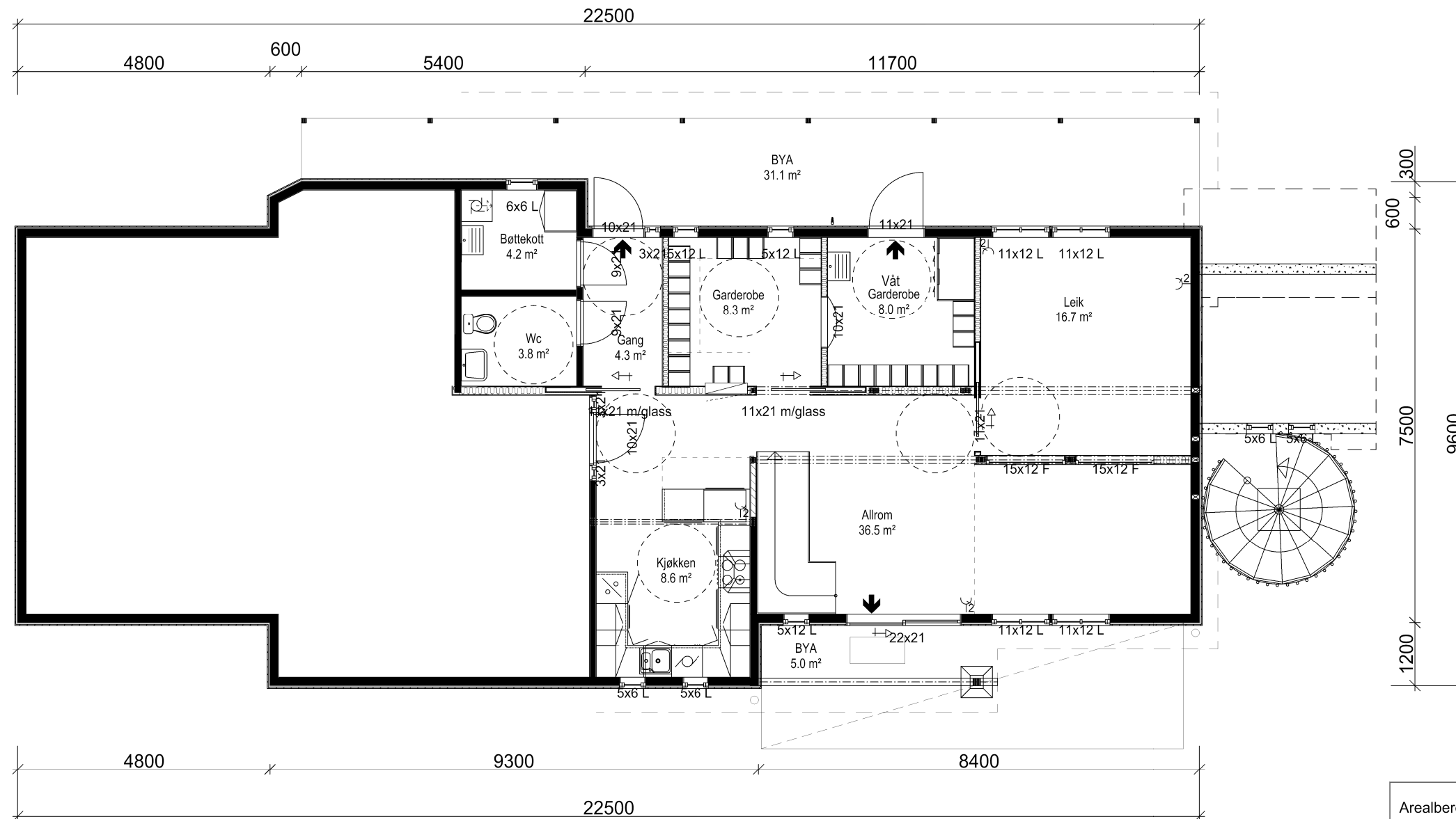
Plan 1. etg - Ny løsning
