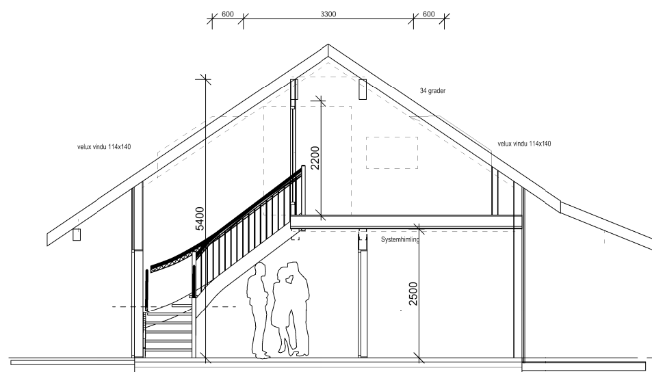
Snitt A-A
