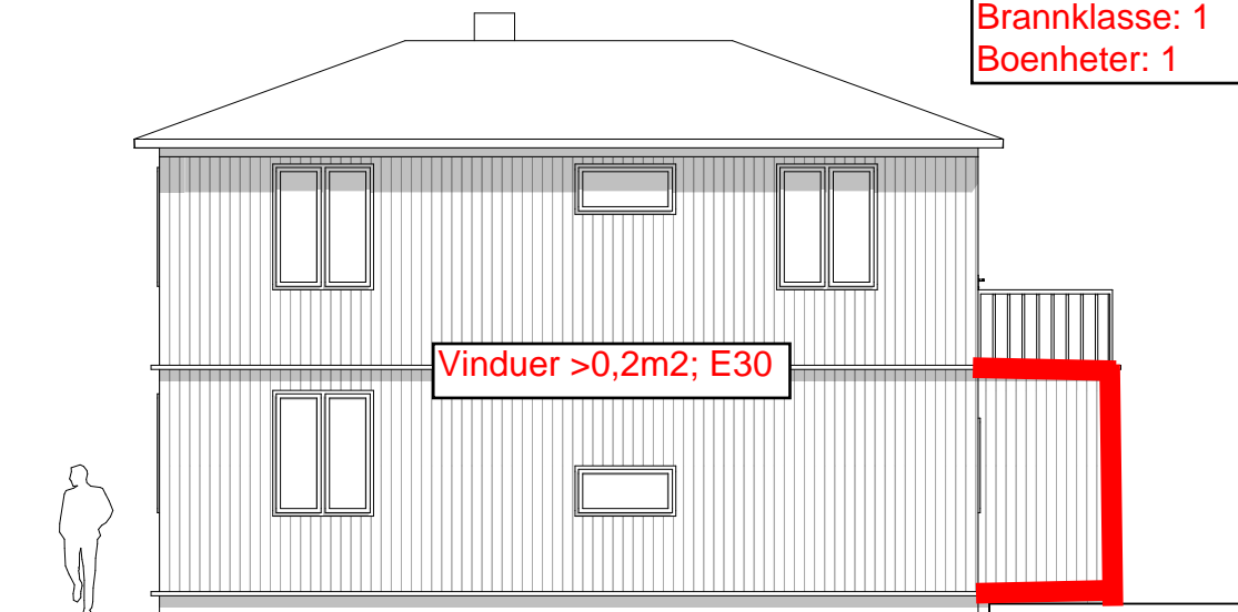
1:100 Fasade ØST
