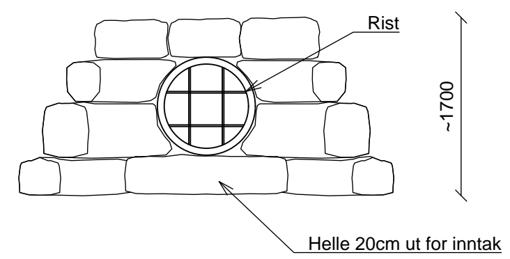
Prinsippskisse vingemur A-A 1:50
