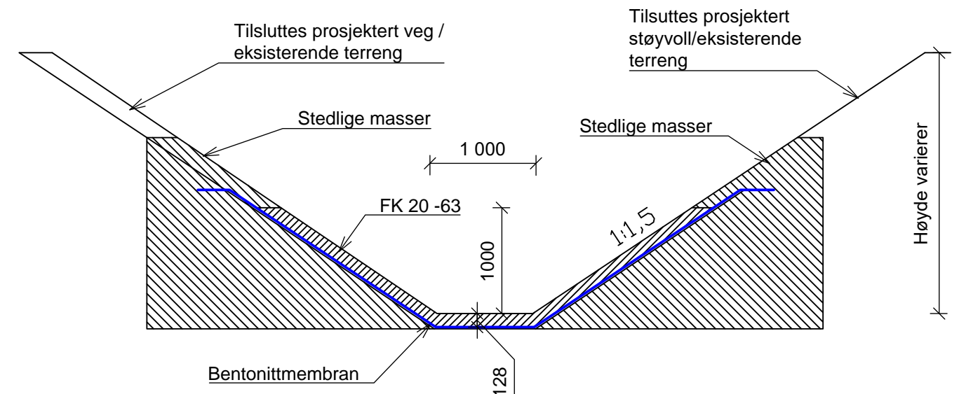
Prinsippskisse Grøft sør for KH4/KH5 1:50
