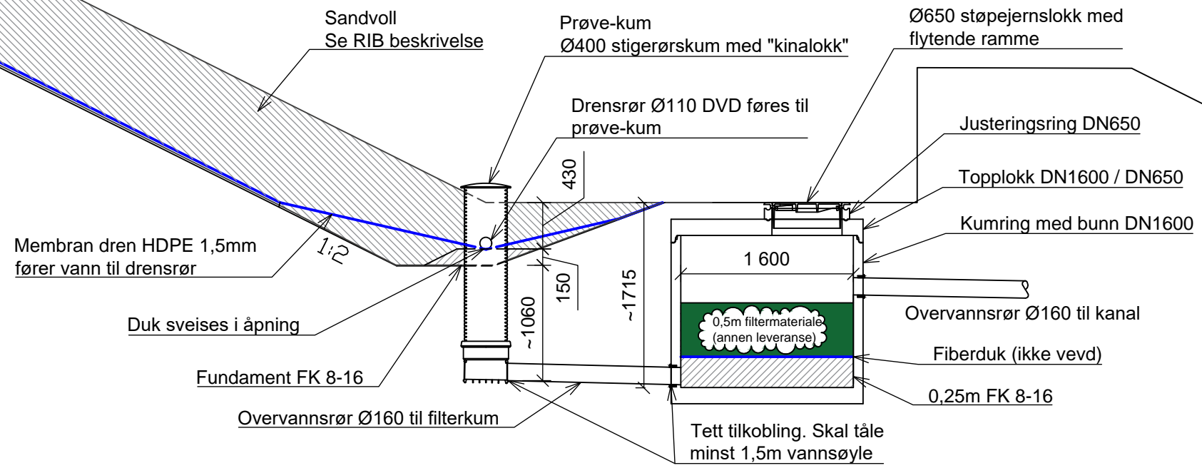
Snitt Drensledning KH4/KH5 og filterkum 1:50
