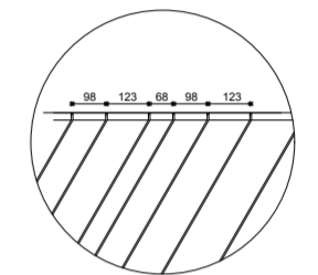
Detalj 2b
