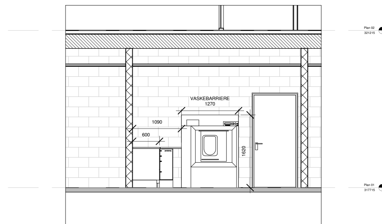
SNITT SKJEMA VASKEROM II 1 : 50
