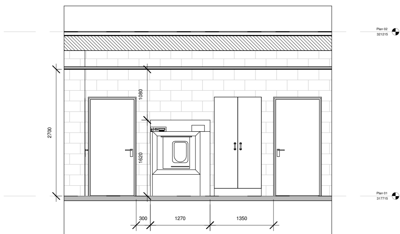
SNITT - SKJEMA VASKEROM 1 : 50
