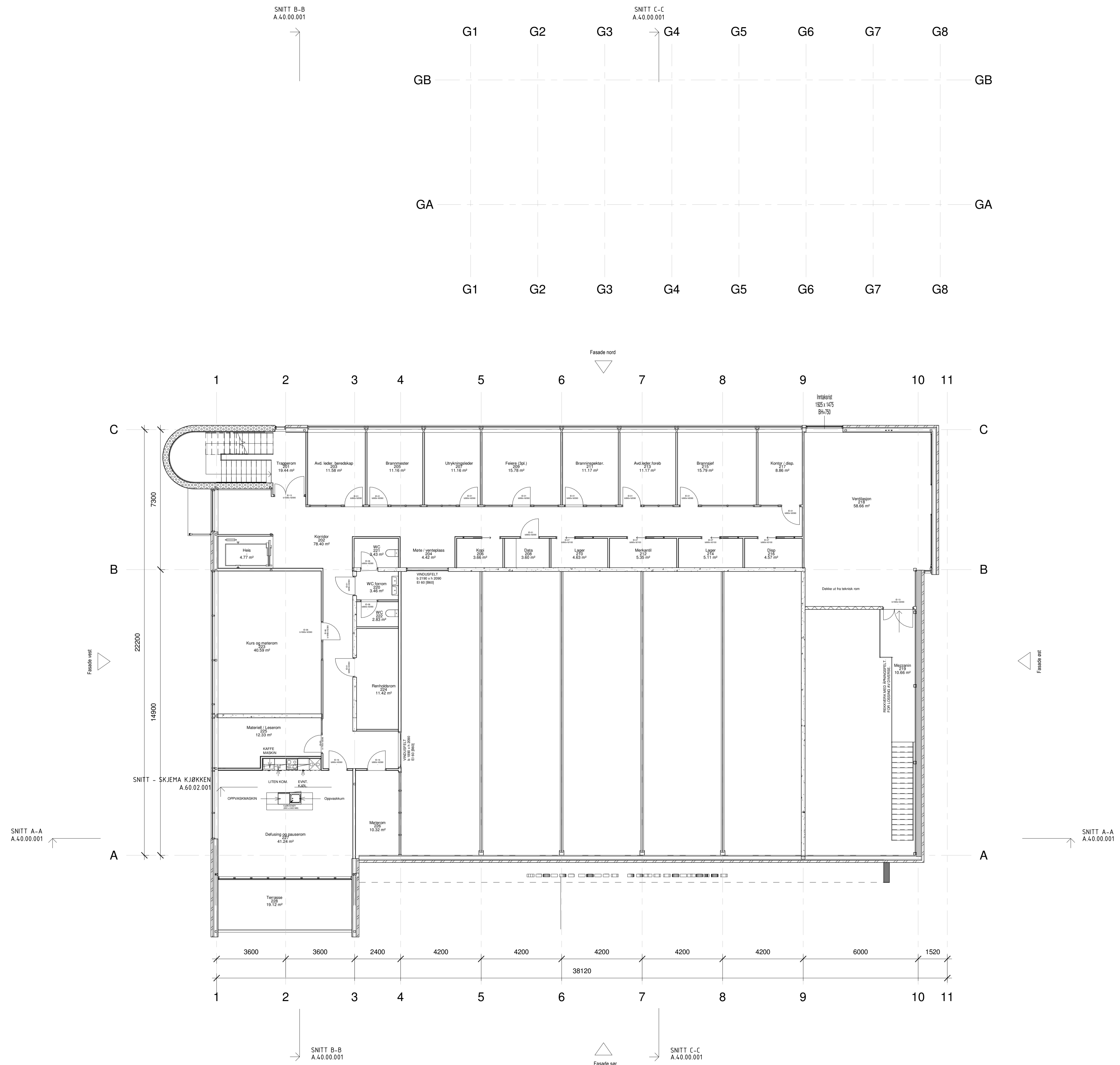
Plan 02 - m/Garasje 1 : 100
