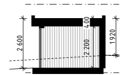
1:200 Snitt E sportsbod
