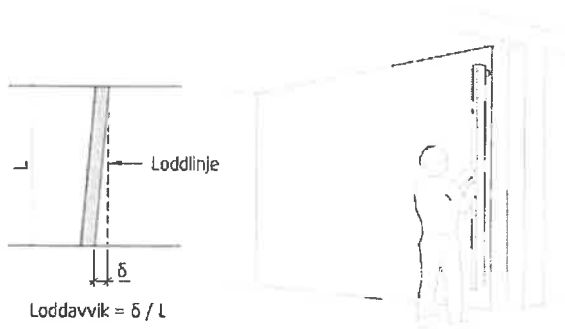
Fig. 42 Måling av loddavvik
