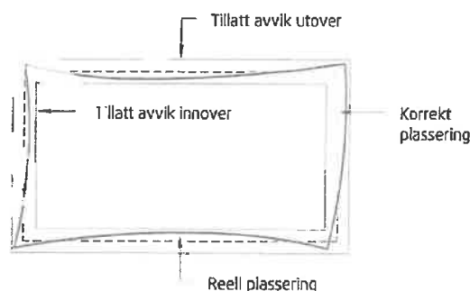
Fig. 61 Plassering i forhold til tillatt sammensatt byggtoleranse
