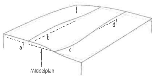
Fig. 33 Total planhet Overflaten er tegnet med heltrukne linjer, mens middelplanet er stiplet. Planhetsavvik i forhold til middelplanet er angitt med a, b, c og d.
