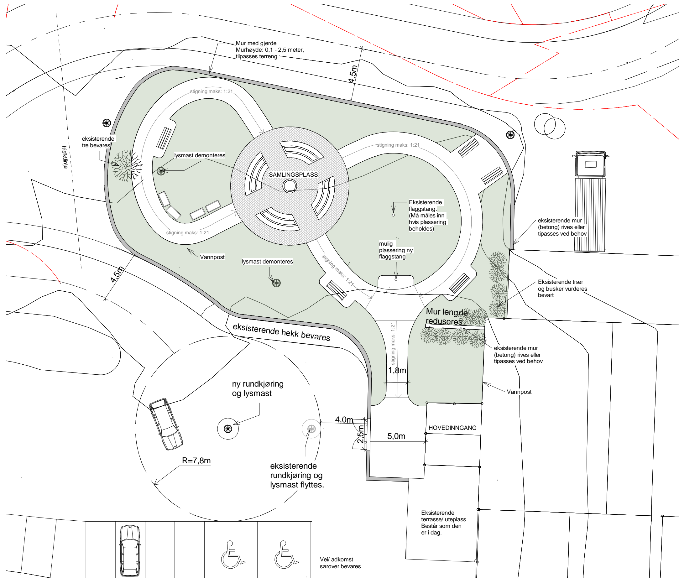
1 Forenkla utomhusplan 1 : 200
